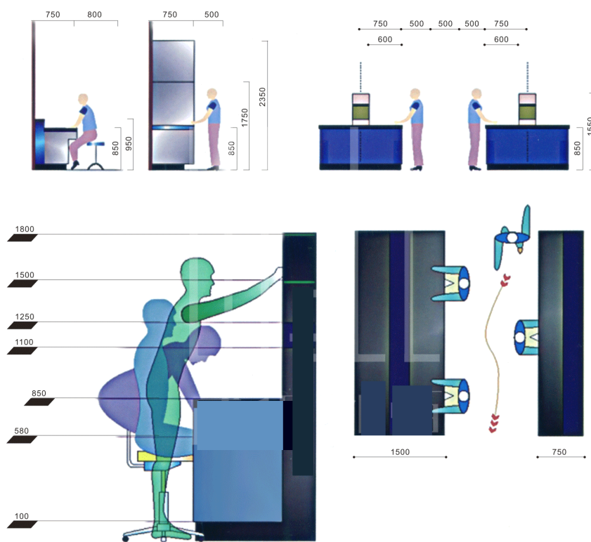
图1-32 室内空间人机关系与尺寸设计
