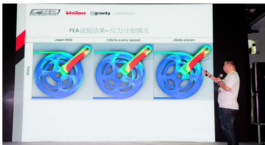
图1-50 应力分布研究
