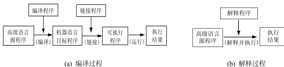
图 1-4 将源程序翻译成机器指令的过程
