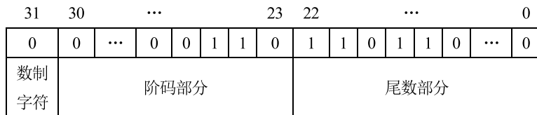
图 1-6 浮点数示例
