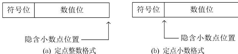
图 1-5 定点数格式
