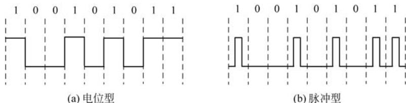
图 3.7 数字信号表示形式
