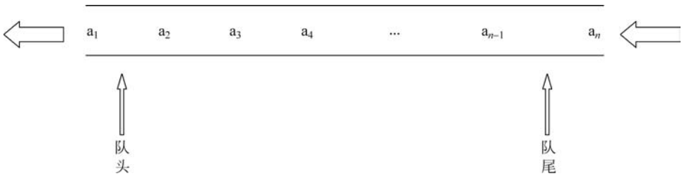
图 3.13 队列示意图
