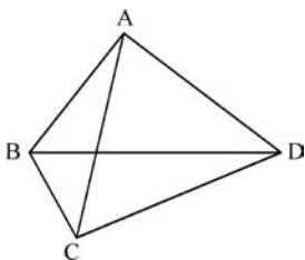
图 3.15 图形结构
