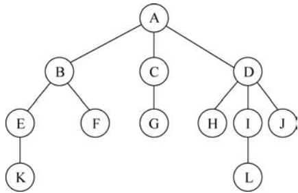
图 3.14 树形结构
