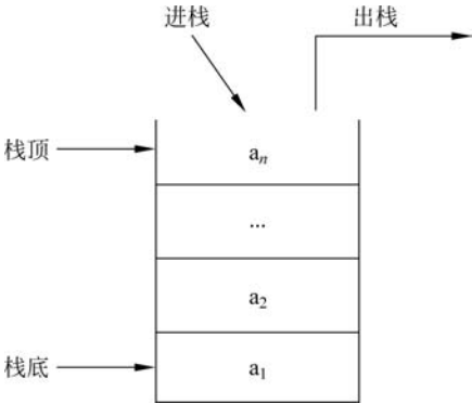
图 3.12 栈的示意图
