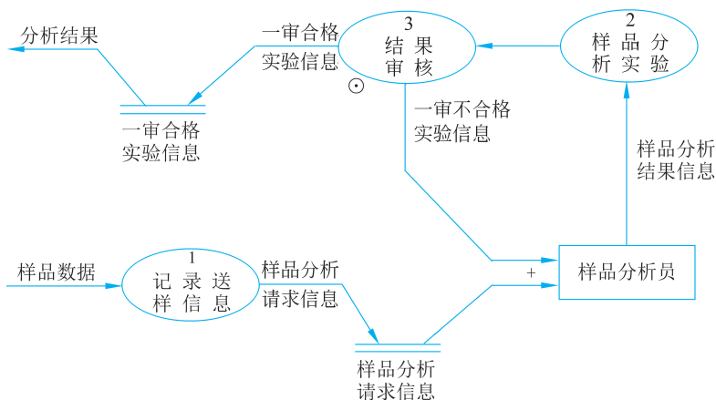
图 3.3 根节点 0 的子节点数据流图
