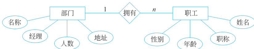
图 3.5 “部门”和“职工”的 E-R 图
