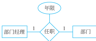
图 3.11 系统 a 的局部 E-R 图
