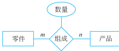
图 3.13 系统 c 的局部 E-R 图
