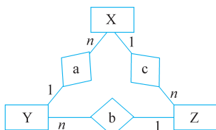
图 3.8 带环结构的 E-R 图
