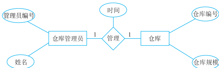
图 3.9 “仓库管理员”和“仓库”的 E-R 图
