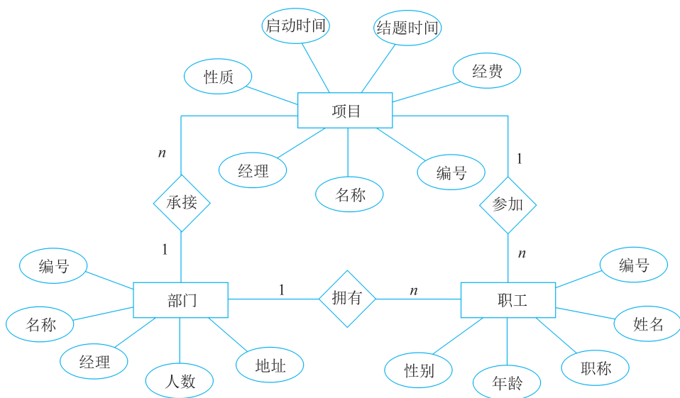
图 3.7 企业信息管理系统的 E-R 图
