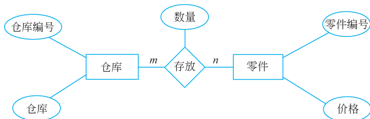
图 3.10 “仓库”和“零件”及其联系的 E-R 图
