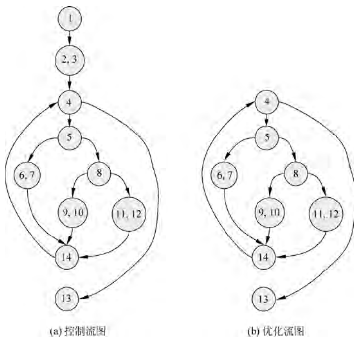
图 5-8 示例程序的控制流图
