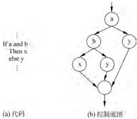
图 5-6 复合逻辑下的控制流图
