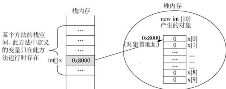
图 5.2 声明数组并分配相应的内存空间, 引用变量指向数组对象
