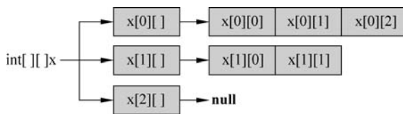
图 5.6 Java 语言中的二维数组可以看成是多个一维数组
