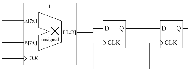
图 5-19 流水线在后的乘法器
