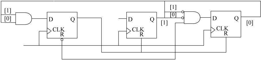
图 5-29 用安全模式状态机实现
