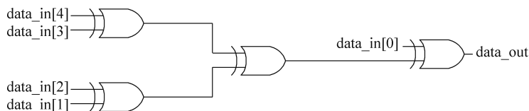
图 5-9 树状结构
