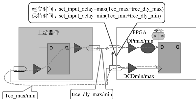
图 5-36 输入端口的时序约束
