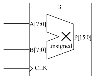
图 5-20 流水线移进乘法器
