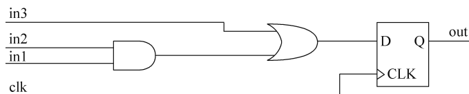
图 5-7 采用阻塞赋值的不正确的实现
