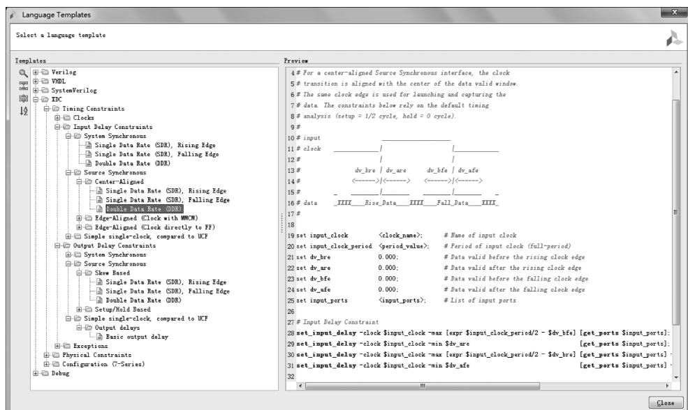
图 5-38 规定 I/O 时序约束的 XDC 模板
