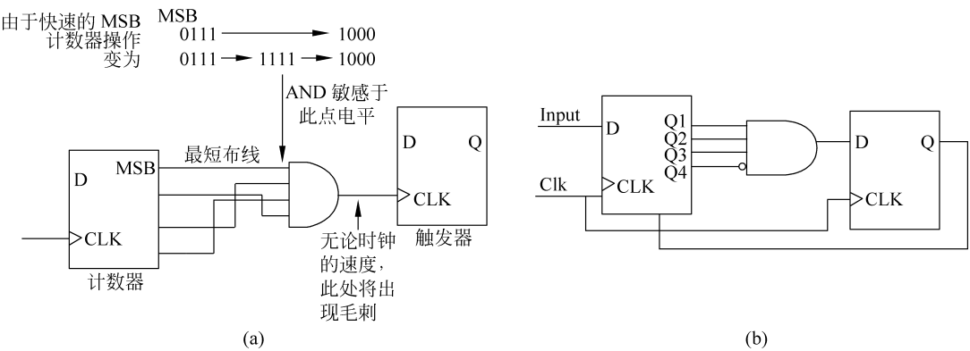
图 5-44 消除产生的毛刺信号
