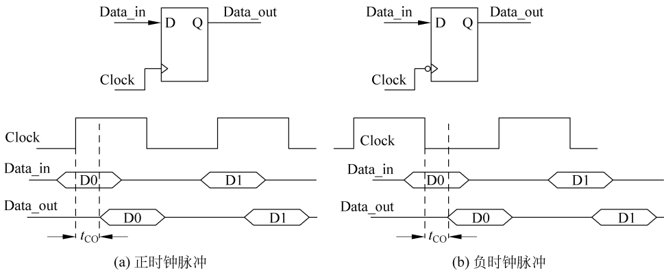
图 5-30 正负时钟脉冲
