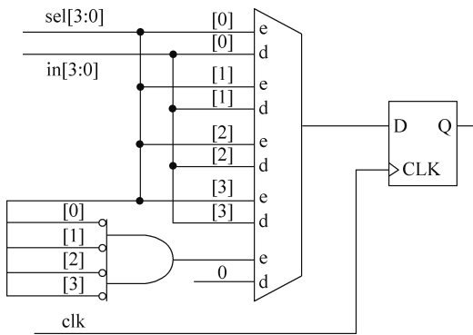
图 5-4 为默认条件编码
