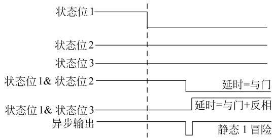
图 5-26 潜在的冒险
