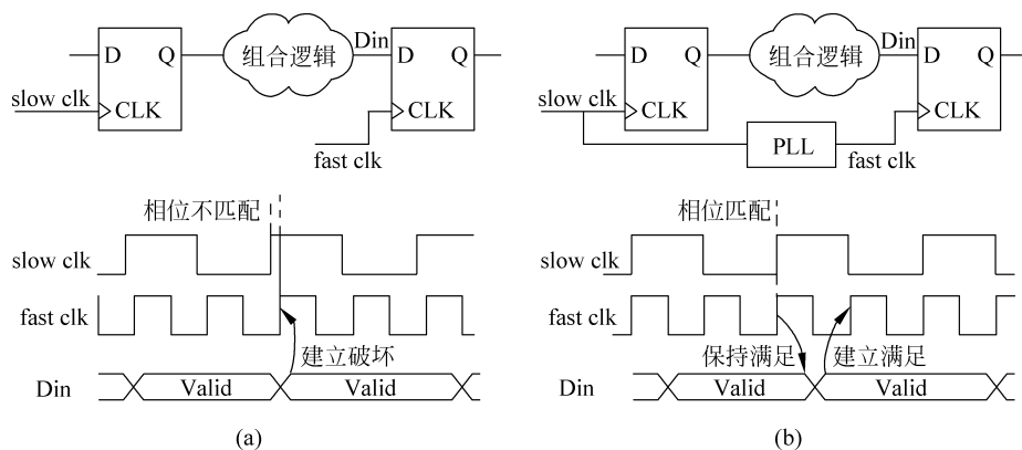
图 5-41 相位控制方法消除亚稳态
