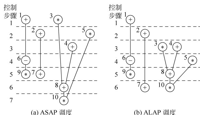
图 5-48 ASAP 和 ALAP 调度的示例
