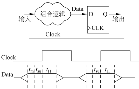
图 5-33 定义建立时间和保持时间
