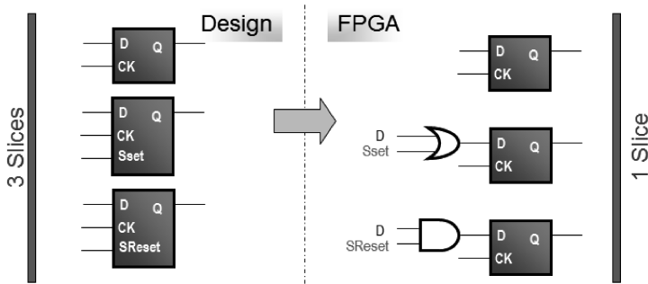
图 5-13 三个不同控制集变为一个相同的控制集
