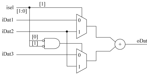
图 5-17 加法器共享时额外的逻辑层次
