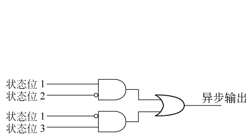
图 5-25 Moore 机输出
