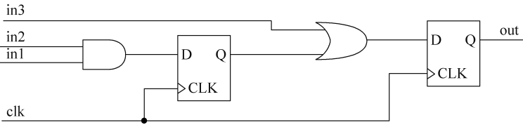
图 5-6 用非阻塞赋值的简单逻辑
