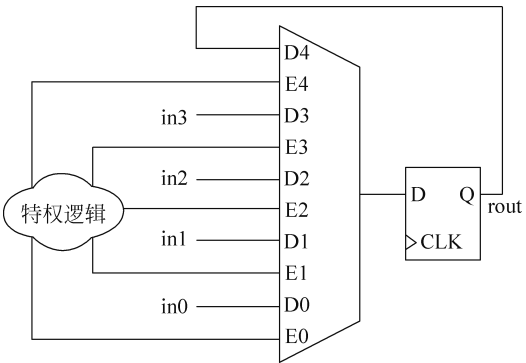
图 5-2 特权多路选择器
