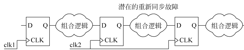
图 5-24 平衡应用于重新同步寄存器
