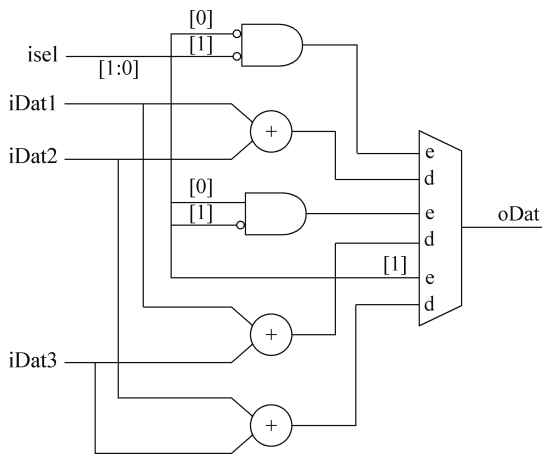
图 5-16 直接映射三个加法器
