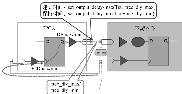
图 5-37 输出端口的时序约束
