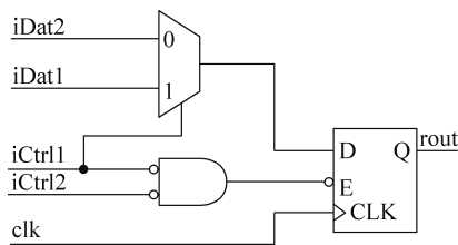
图 5-5 带明显特权的实现
