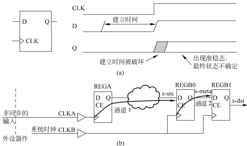
图 5-39 准稳态的产生和消除
