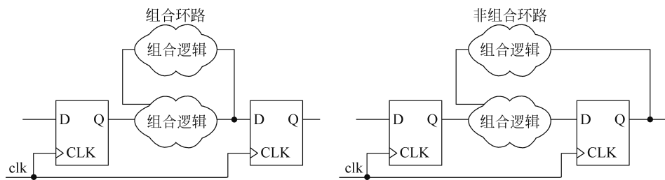
图 5-10 组合与时序环路
