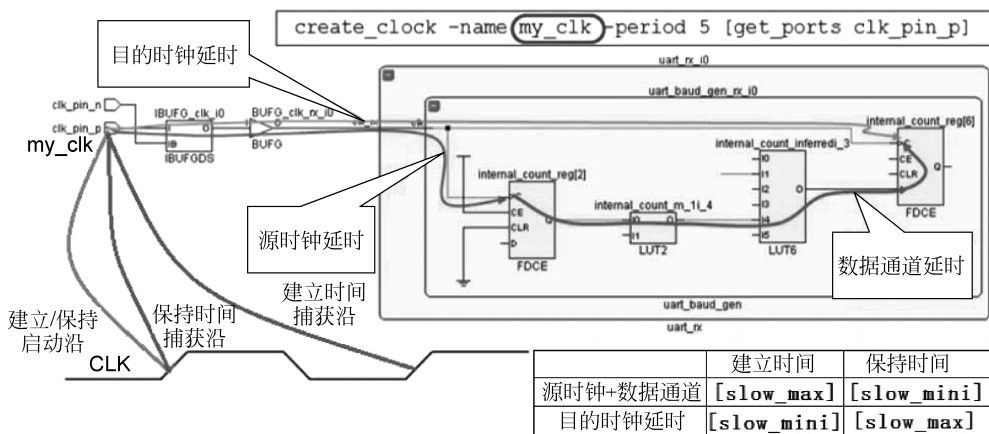
图 5-35 建立和保持时间的三条路径延时
