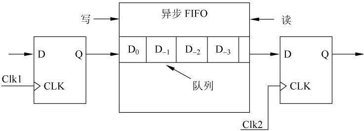
图 5-42 异步 FIFO
