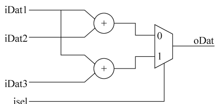
图 5-14 两个加法器的直接实现
