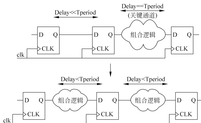
图 5-18 平衡组合逻辑
