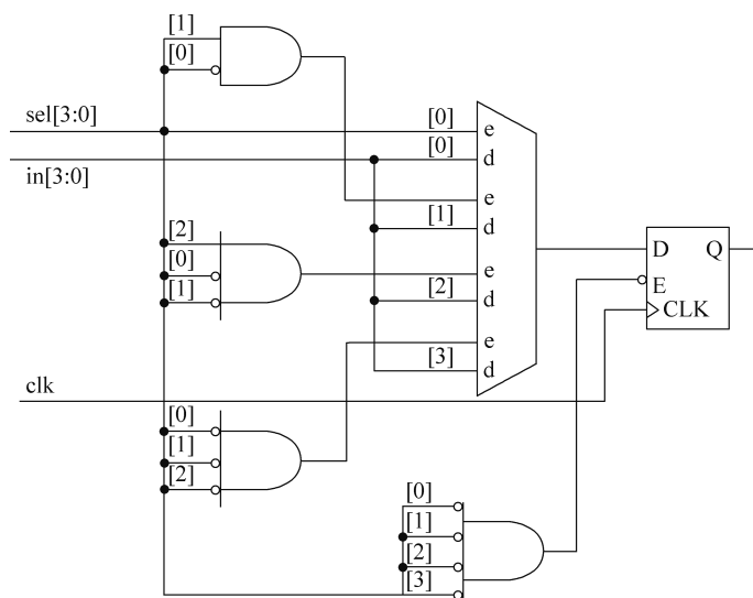
图 5-3 特权译码逻辑
