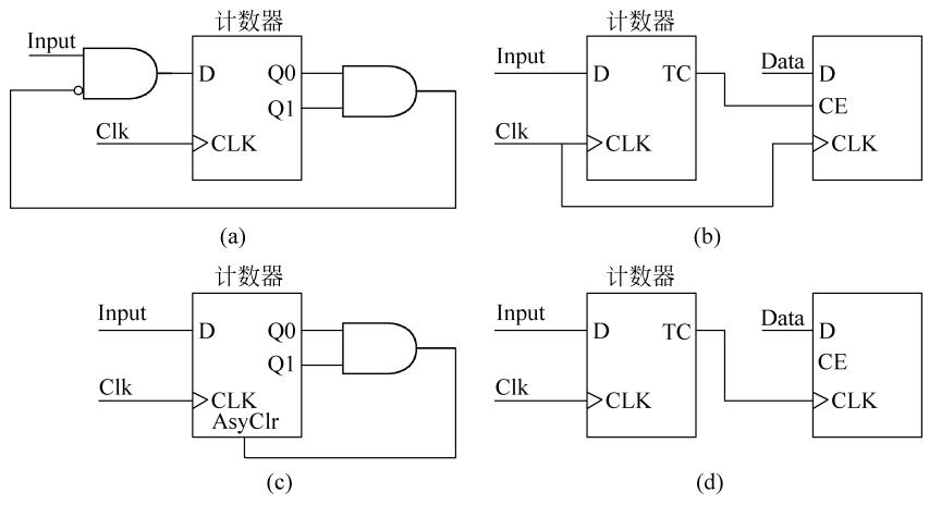
图 5-45 同步设计示例(a)(b)以及异步设计示例(c)(d)
