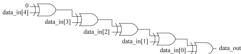
图 5-8 链状结构
