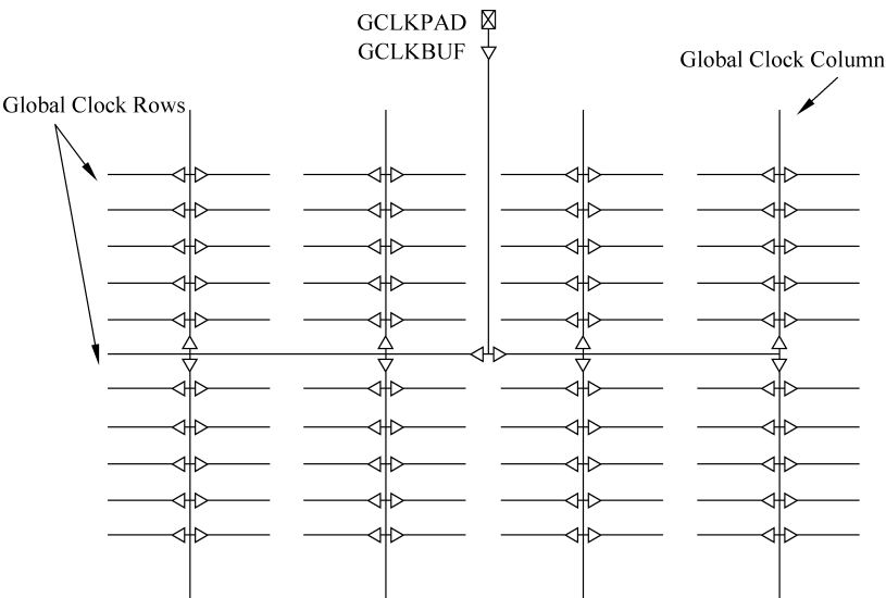
图 5-31 典型的时钟分配网络
