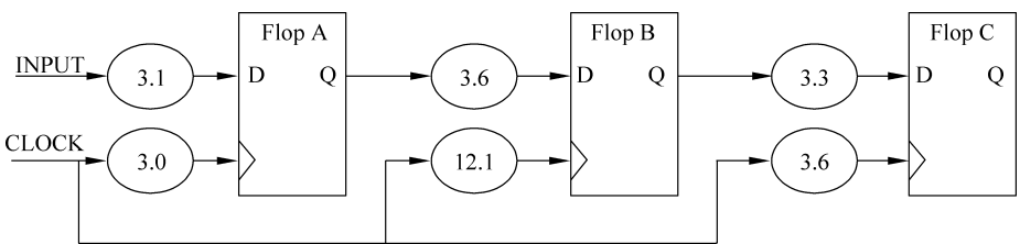
图 5-40 时钟相位偏移影响触发器正常工作
