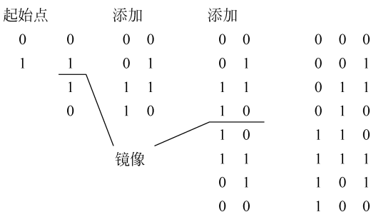
图 5-27 产生格雷码
