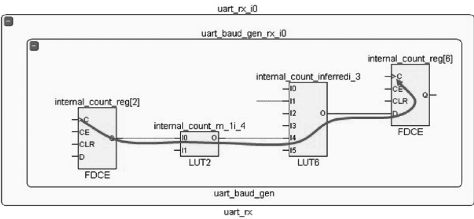
图 5-34 同步设计中的静态时序通道
