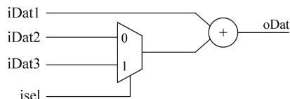
图 5-15 组合加法器资源
