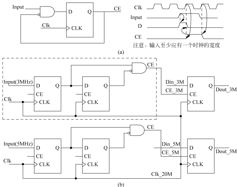
图 5-43 生成时钟使能信号
