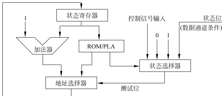
图 5-49 基本的控制器结构
