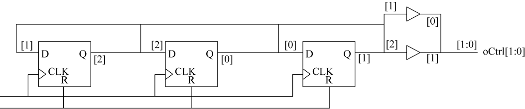
图 5-28 简单的状态机实现
