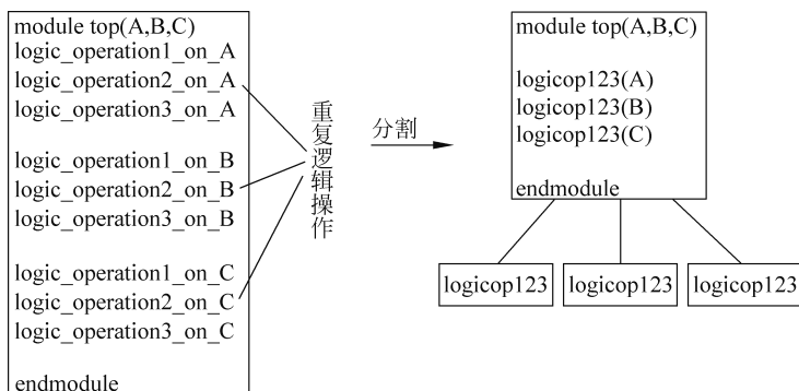
图 5-12 模块设计
