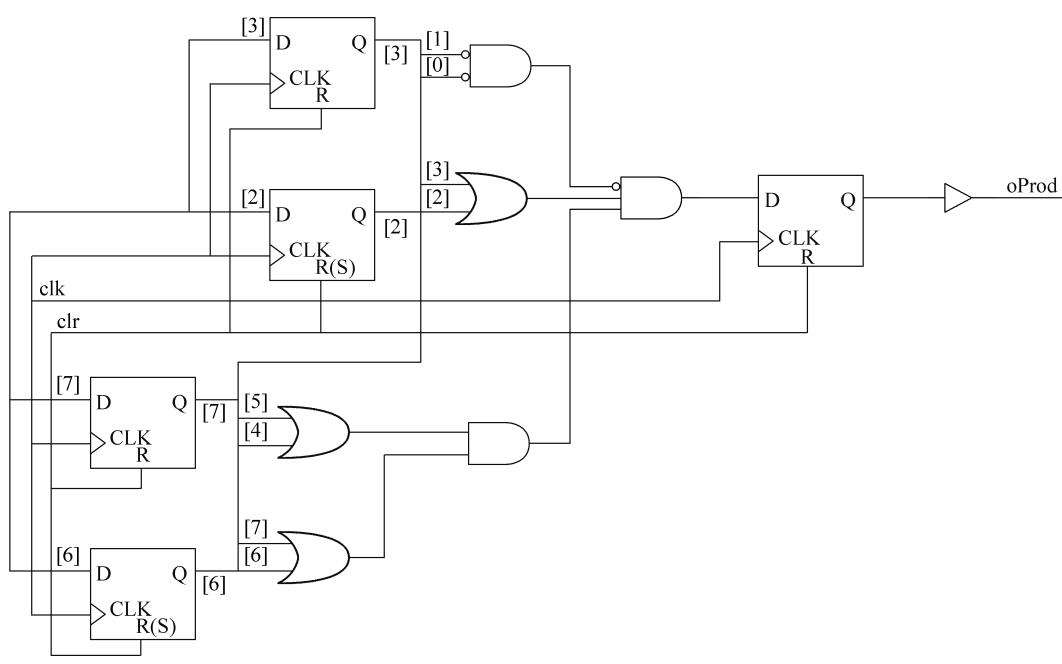
图 5-21 不平衡的逻辑
