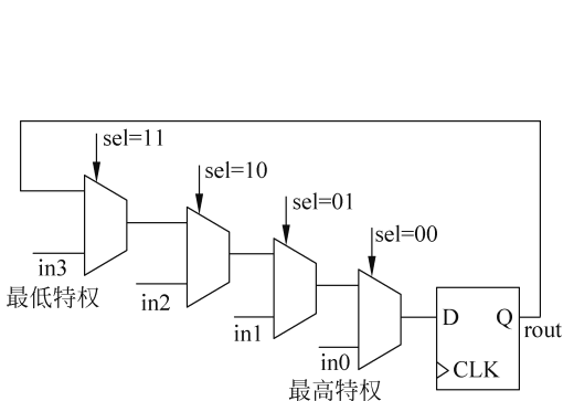
图 5-1 串行多路选择器结构的简单特权
