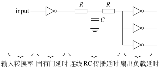
图 5-32 元件产生延时的四个分量
