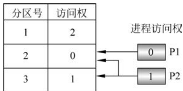
图 3.7 访问授权保护法
