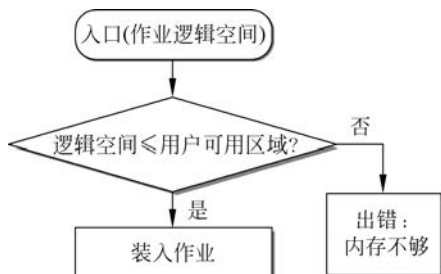
图 3.9 单一分区分配流程
