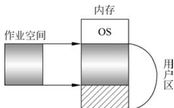
图 3.8 单一分区
