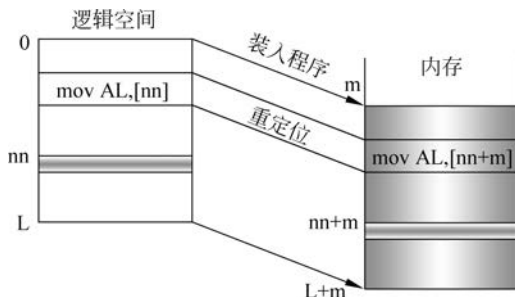
图 3.4 静态重定位
