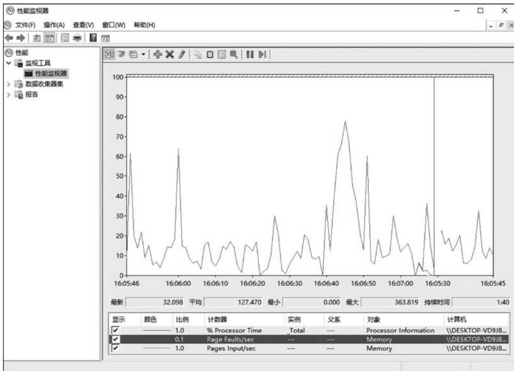
图 3.2 页面在内存中换出换进
