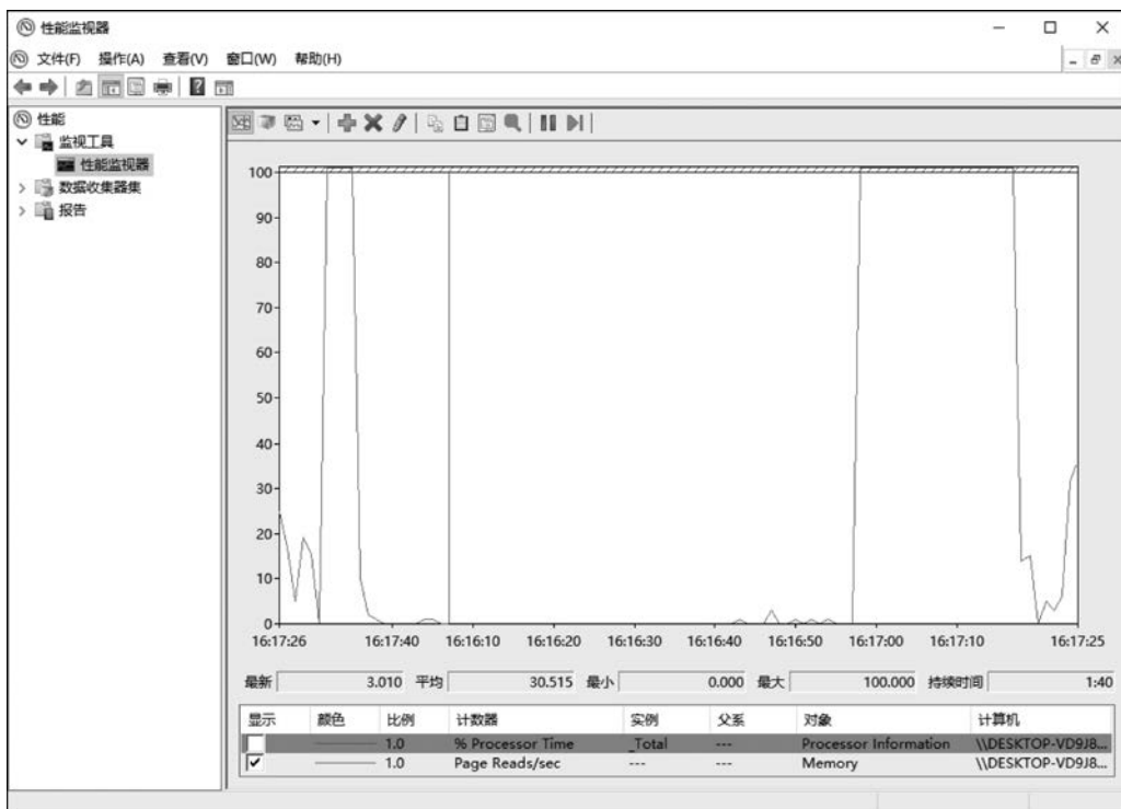
图 3.30 Windows 10 缺页次数变化
