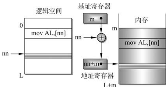
图 3.5 动态重定位
