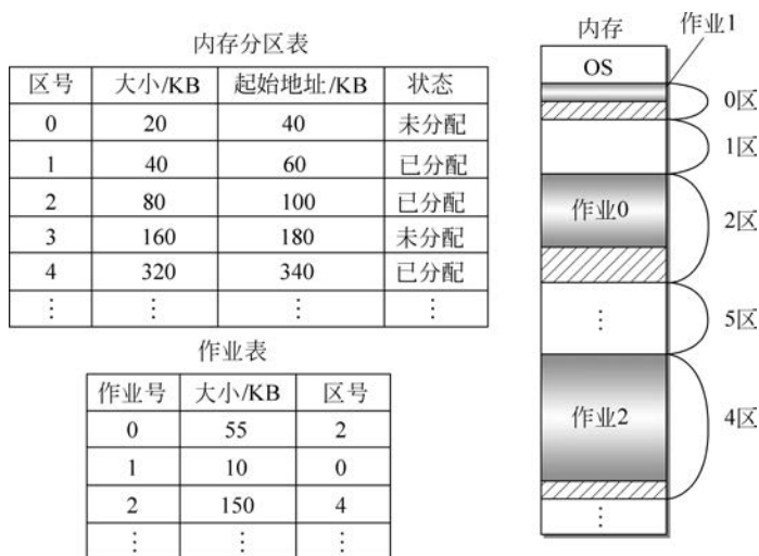
图 3.10 多重固定分区
