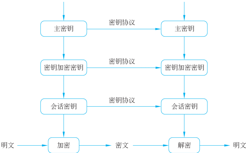
图 3.2 三级密钥管理的层次结构
