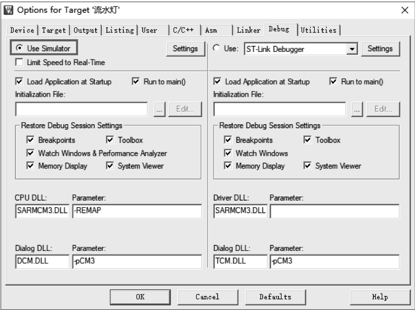
图 3-7 Debug 选项卡
