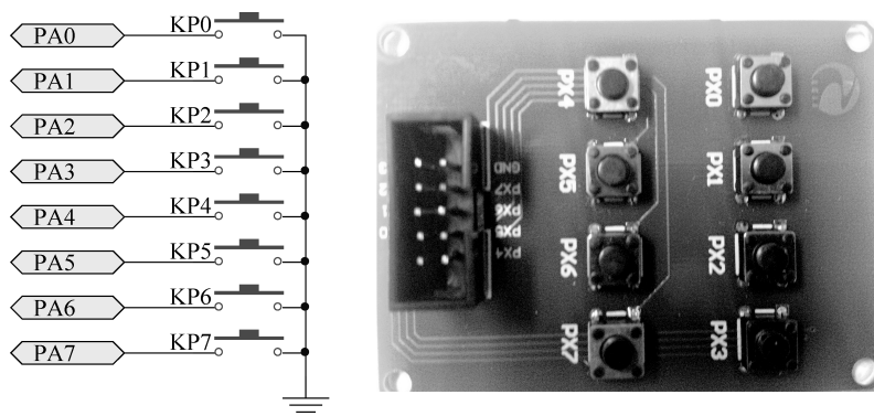
图 3-16 按键电路图
