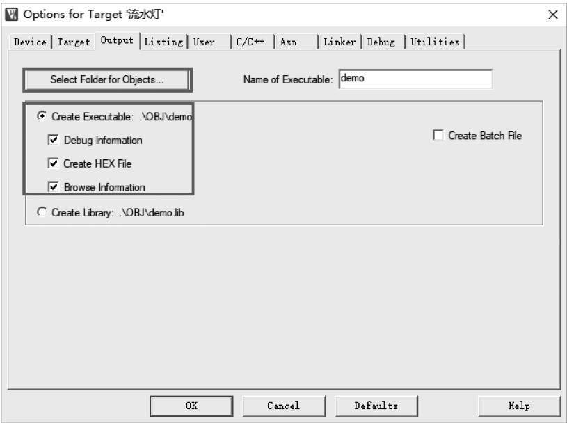
图 3-4 Output 选项卡
