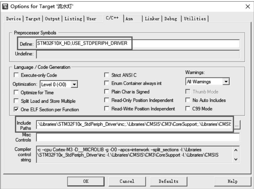
图 3-6 C/C++选项卡
