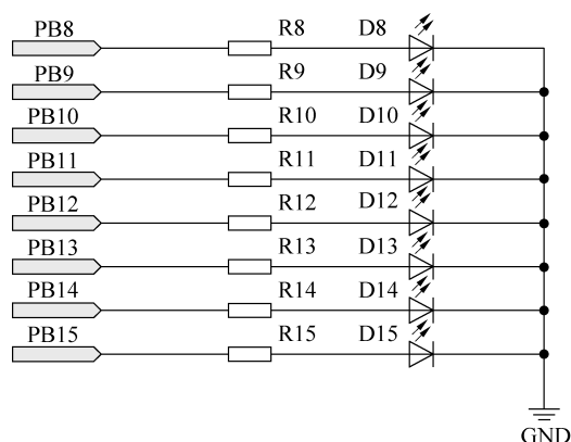
图 3-8 流水灯电路
