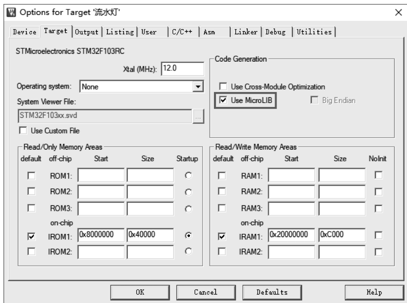
图 3-3 Target 选项卡
