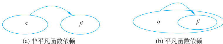
图 5-5 非平凡函数依赖及平凡函数依赖图
