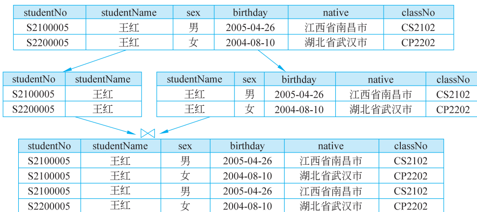
图 5-2 有损分解举例
