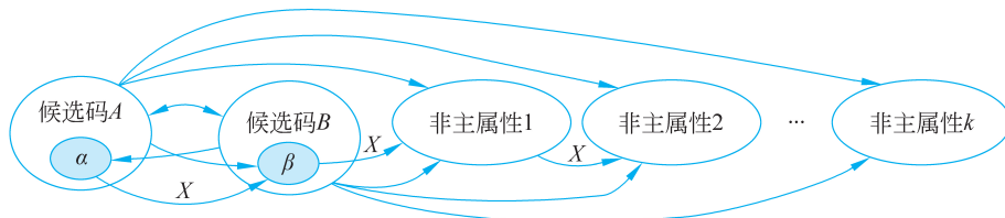
图 5-10 BCNF 关系模式中的函数依赖
