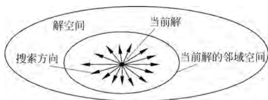
图 3-13 局部搜索的分散性
