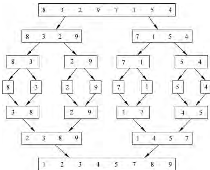
图 3-5 合并排序过程示意图
