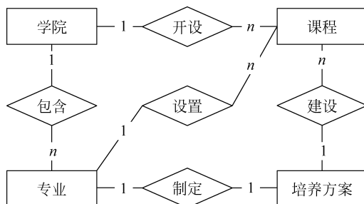
图 5-15 专业建设模块 E-R 图
