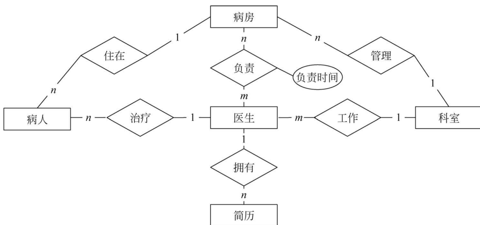
图 5-31 系统总 E-R 图
