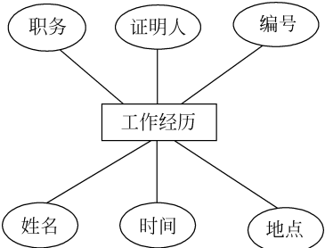
图 5-24 “工作经历”实体及属性
