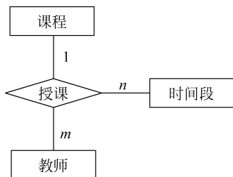
图 5-16 教师授课 E-R 图
