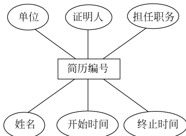
图 5-28 “简历”实体及属性
