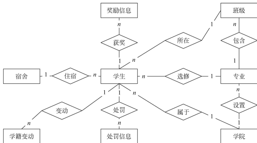
图 5-14 集成后的学籍管理模块的 E-R 图
