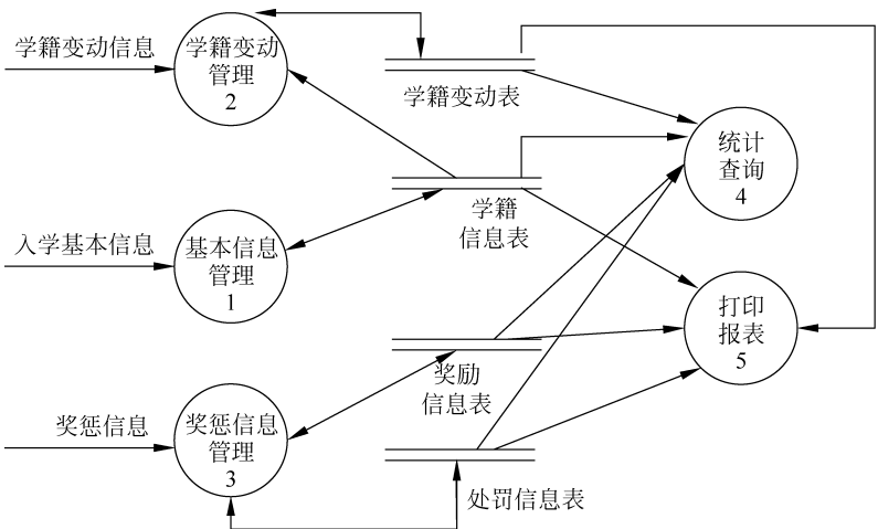
图 5-6 学籍管理子系统的 0 层数据流图
