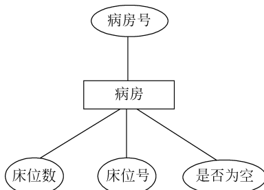
图 5-30 “病房”实体及属性
