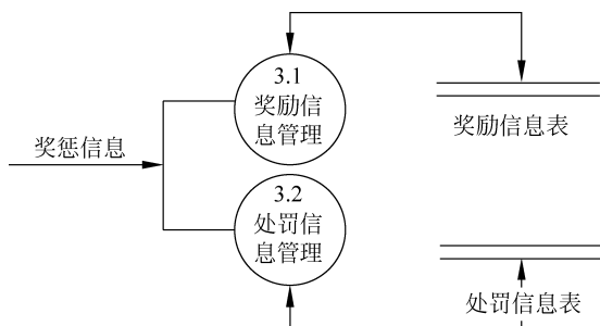
图 5-9 奖惩信息管理一层数据流图
