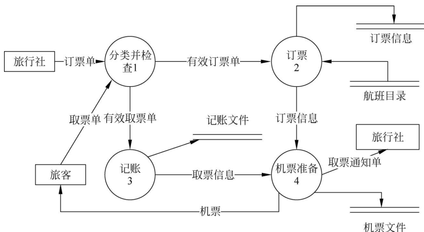
图 5-2 飞机机票预订系统的数据流图
