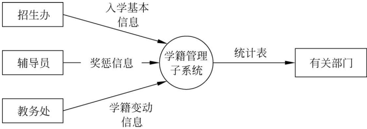
图 5-5 学籍管理子系统的顶层数据流图
