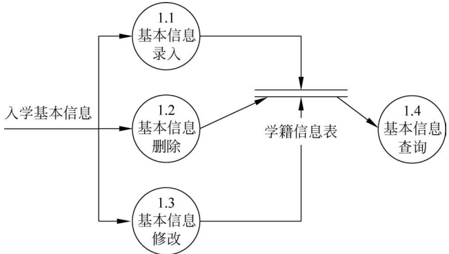
图 5-7 基本信息管理一层数据流图
