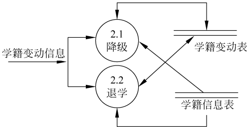
图 5-8 学籍变动管理一层数据流图
