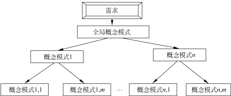
图 5-10 集中式模式设计法的设计过程
