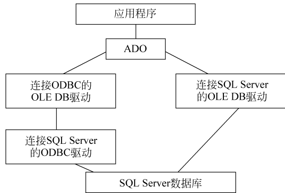
图 5-20 通过 ADO 访问 SQL Server 数据库的接口
