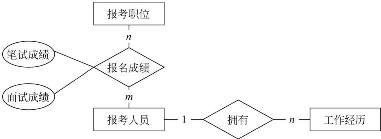
图 5-25 实体之间的联系图
