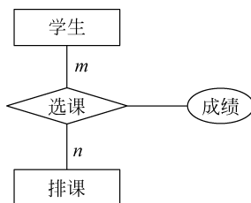
图 5-18 学生选课 E-R 图
