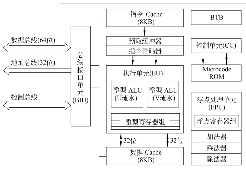
图 3.10 Pentium 处理器的内部结构
