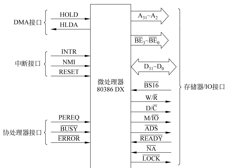
图 3.15 80386 DX 引脚信号分组
