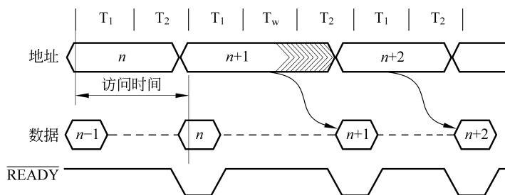
图 3.19 带等待状态的流水线总线周期时序
