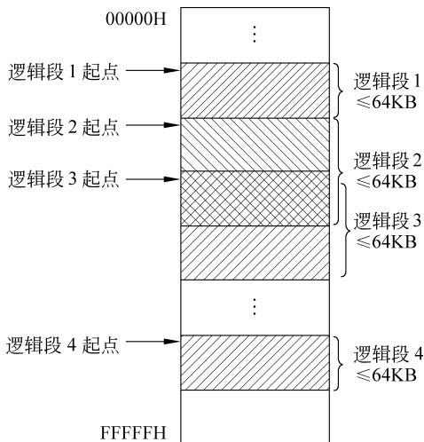
图 3.4 逻辑段在物理存储器中的位置
