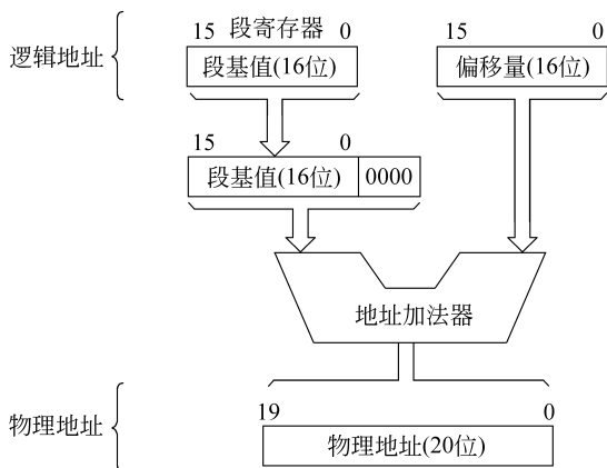
图 3.6 实模式下物理地址的产生
