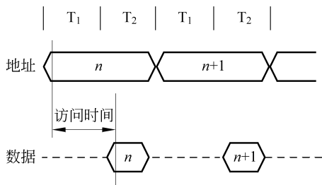
图 3.17 典型的“非流水线总线周期”时序
