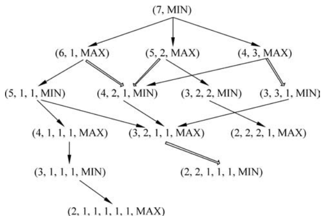
图 3.23 分钱币的博弈
