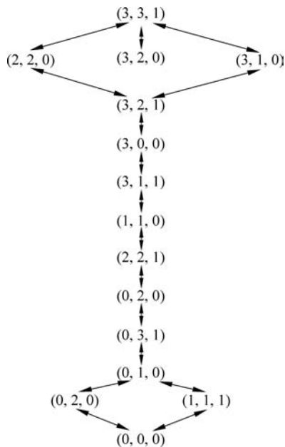
图 3.3 渡河问题的状态空间有向图
