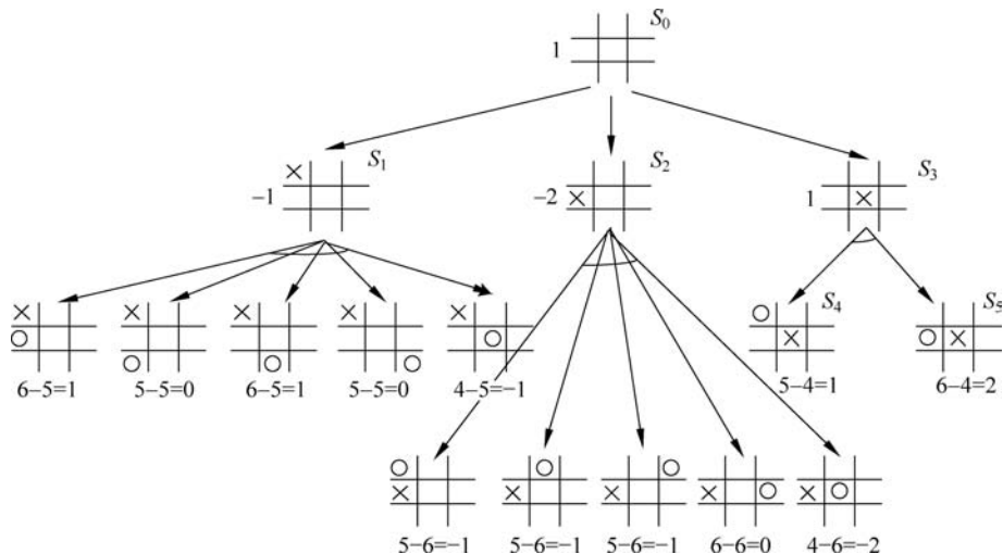
图 3.28 一字棋极大极小搜索
