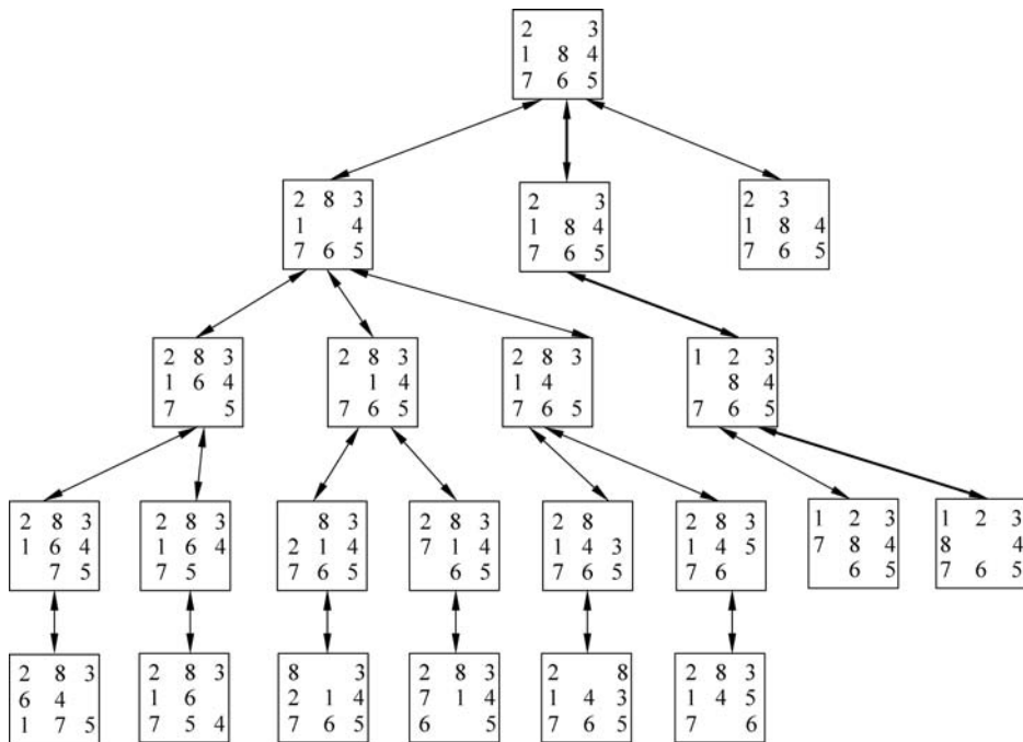
图 3.6 八数码问题的一次搜索图
