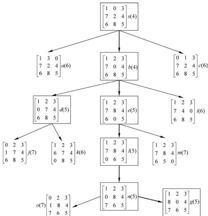
图 3.13 应用 A 算法的八数码搜索图
