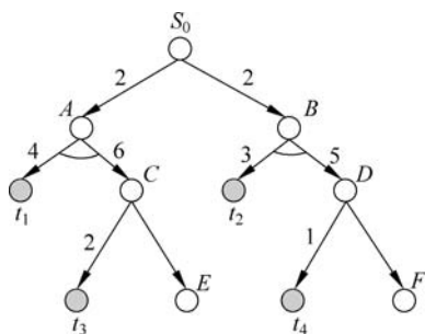
图 3.20 与或树的代价
