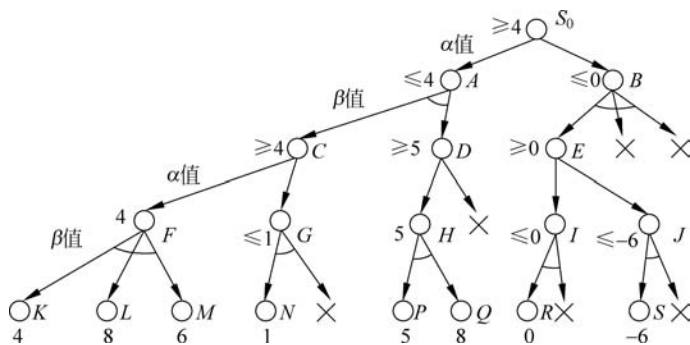
图 3.29 一个 \alpha - \beta 剪枝的具体例子
