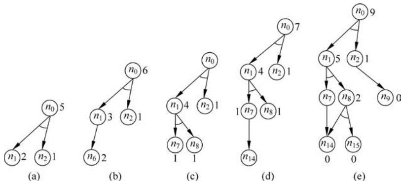
图 3.22 算法 AO^* 搜索过程中解图的形成
