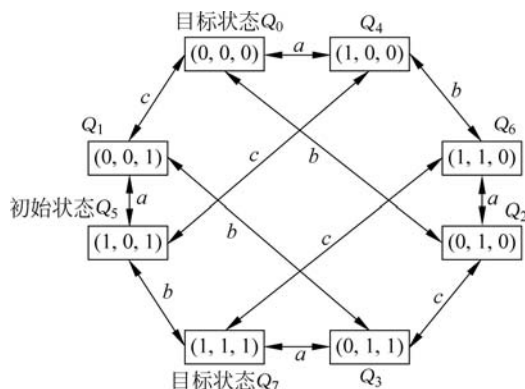
图 3.1 三枚钱币问题的状态空间图
