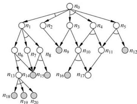
图 3.17 与或图简例
