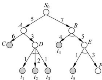
图 3.34 与或树
