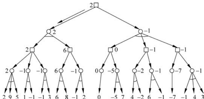
图 3.24 四层博弈树
