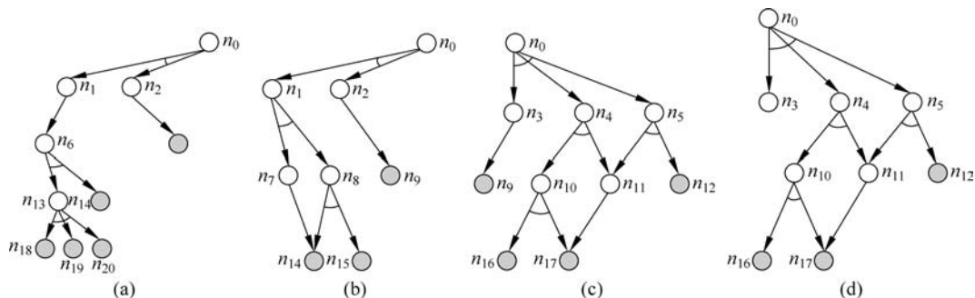
图 3.18 四个可能的解图
