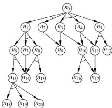
图 3.21 结点编号后的与或图
