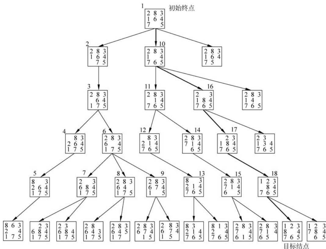
图 3.11 深度优先搜索解决八数码问题
