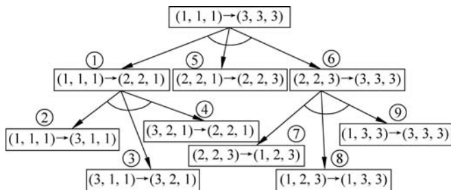
图 3.16 梵塔问题的状态空间图表示
