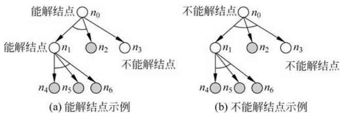
图 3.19 能解结点和不能解结点
