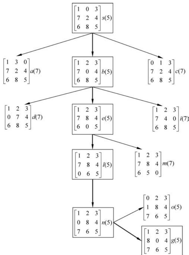
图 3.14 应用启发式函数 p(x) 的八数码问题搜索图
