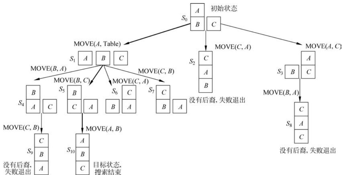
图 3.9 积木问题的宽度优先搜索树
