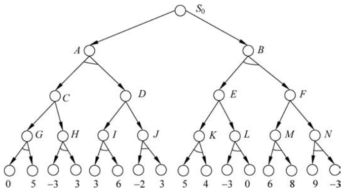
图 3.35 博弈树
