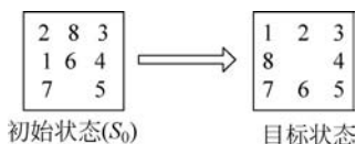
图 3.32 八数码问题
