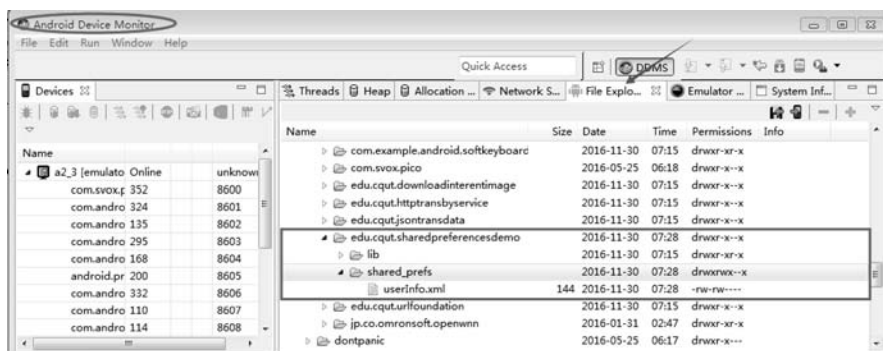
图 5.2 userInfo.xml 文件
