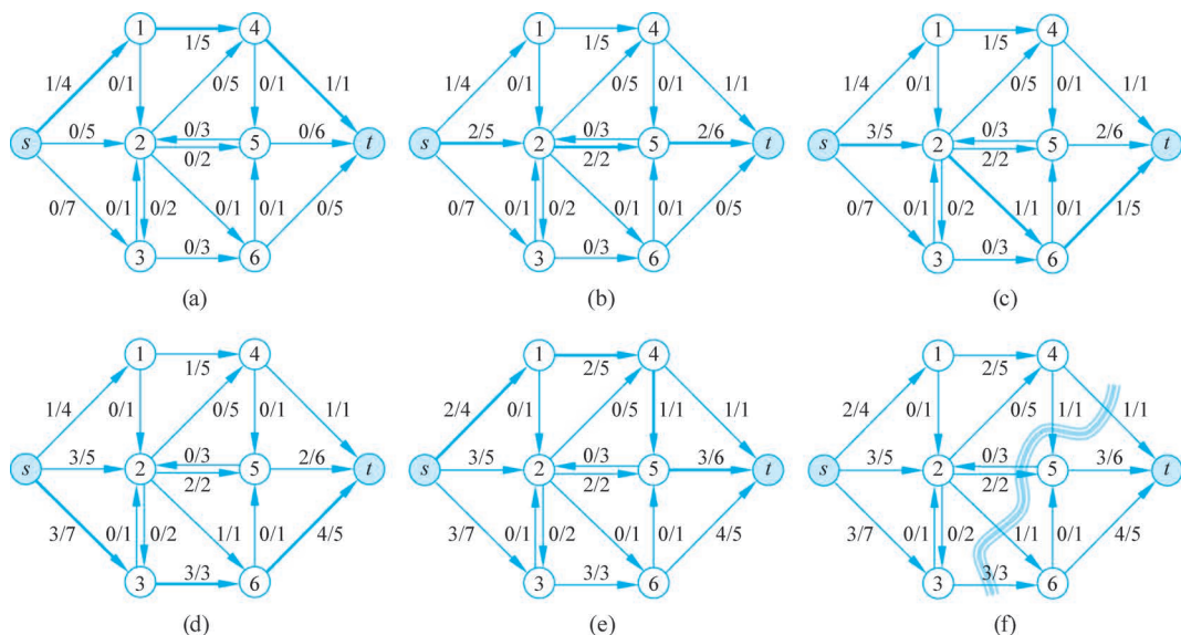
图 3.2.4 增强通路算法计算过程
