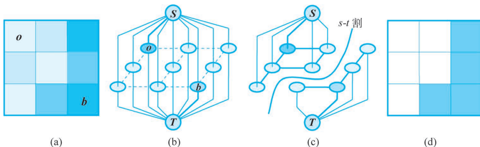
图 3.2.1 图割分割示意图
