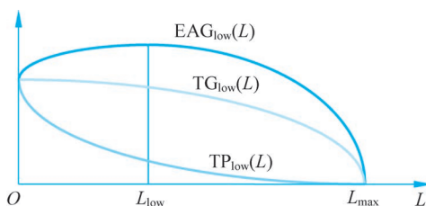
图 3.3.2 对 \text{EAG}_{\text{low}}(L) 曲线是单峰曲线的解释
