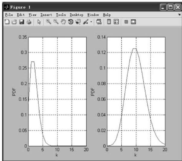
图 5-14 泊松分布 PDF 曲线图
