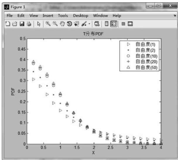
图 5-5 不同自由度定义下的 T 分布 PDF 示意图
