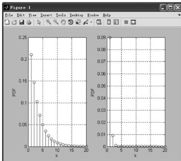
图 5-13 几何分布 PDF
