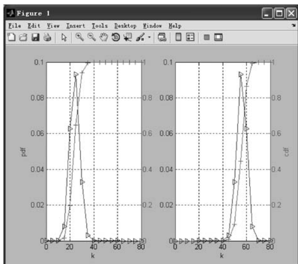
图 5-12 二项分布 PDF 描述曲线图
