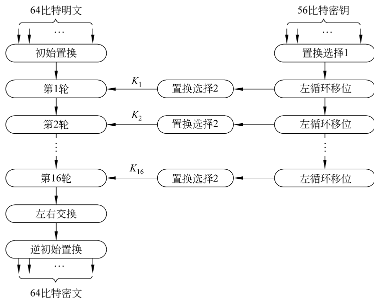
图 3-5 DES 加密算法框图
