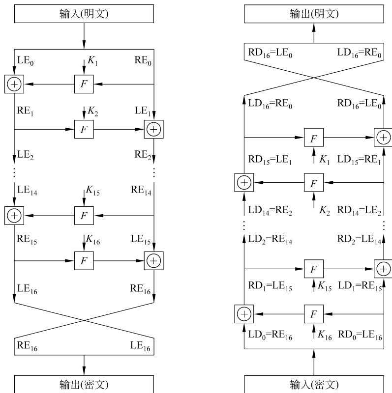
图 3-4 Feistel 加解密过程
