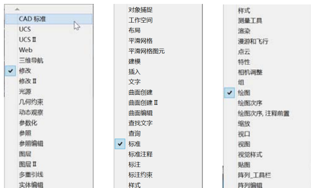
图 2-9 工具栏列表
