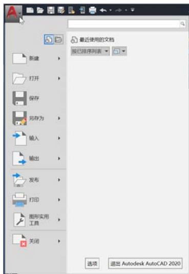
图 2-12 菜单浏览器
