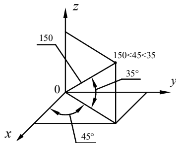
图 2-14 球坐标
