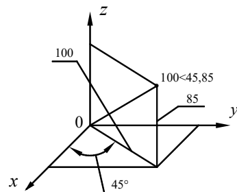
图 2-15 柱坐标
