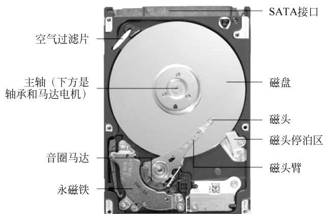
图 1-10 机械硬盘
