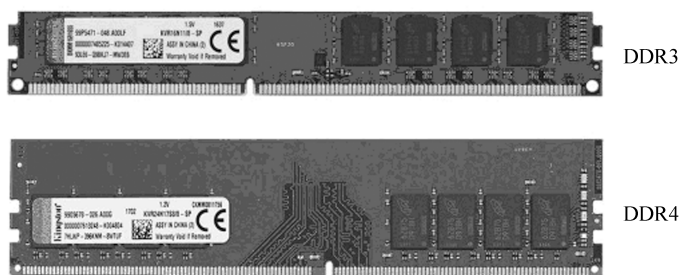
图 1-9 内存条
