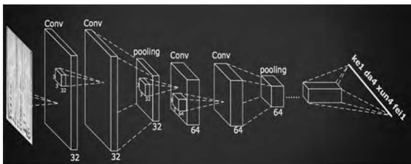
图 5.16 DFCNN 示意图
