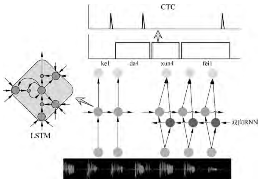
图 5.15 基于 RNN-CTC 的主流语音识别系统框架
