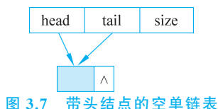
图 3.7 带头结点的空单链表
