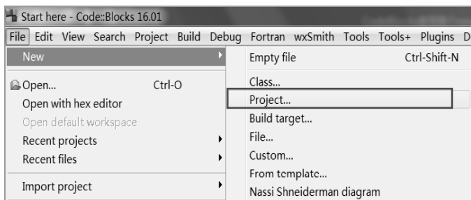
图 1-10 创建新工程
