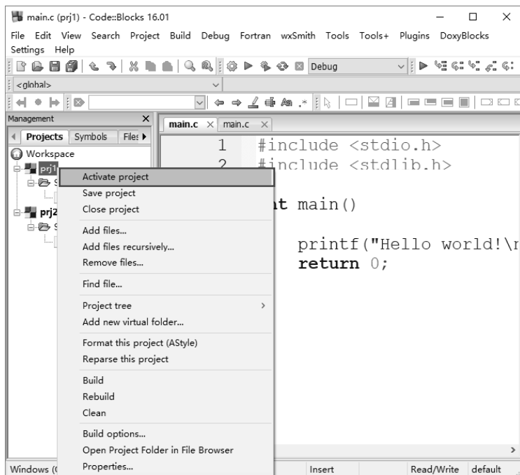
图 1-22 激活工程
