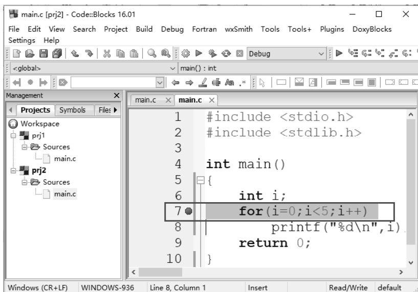
图 1-24 设置断点
