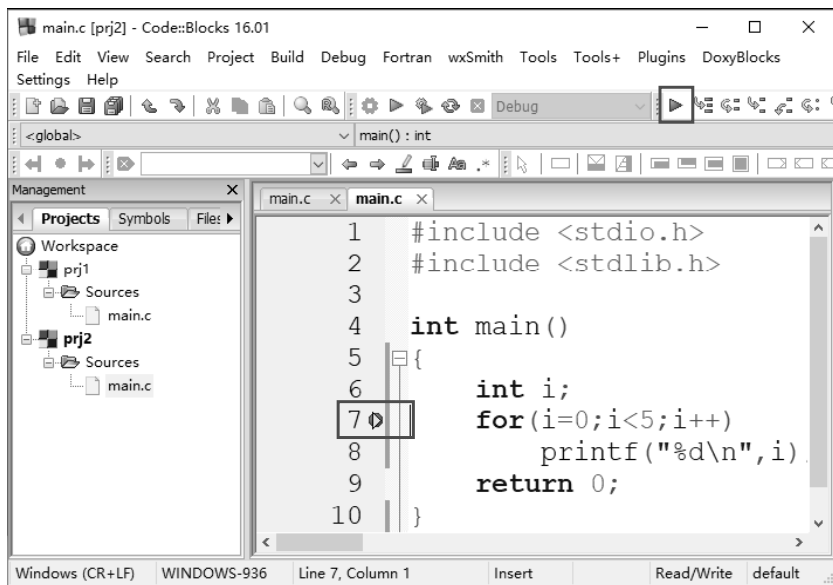
图 1-25 开始调试
