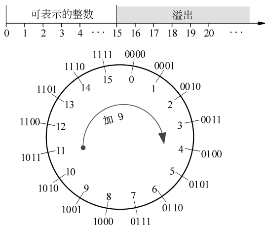
图 3-2 无符号整数的溢出
