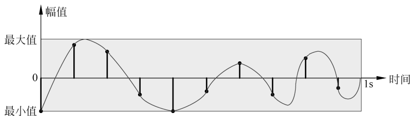
图 3-8 音频信号的采样
