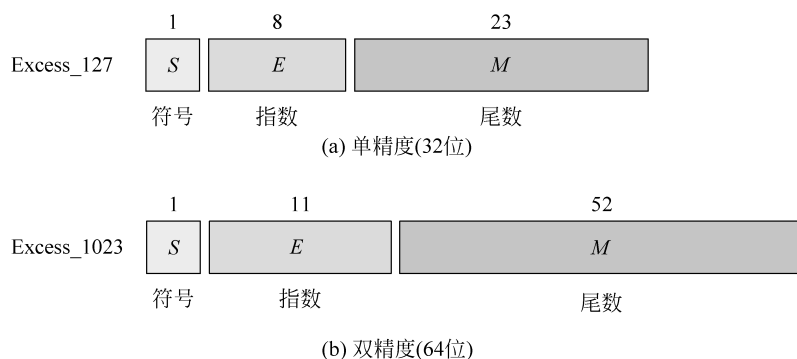
图 3-7 IEEE 单精度和双精度表示
