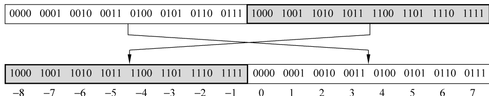
图 3-4 补码表示法
