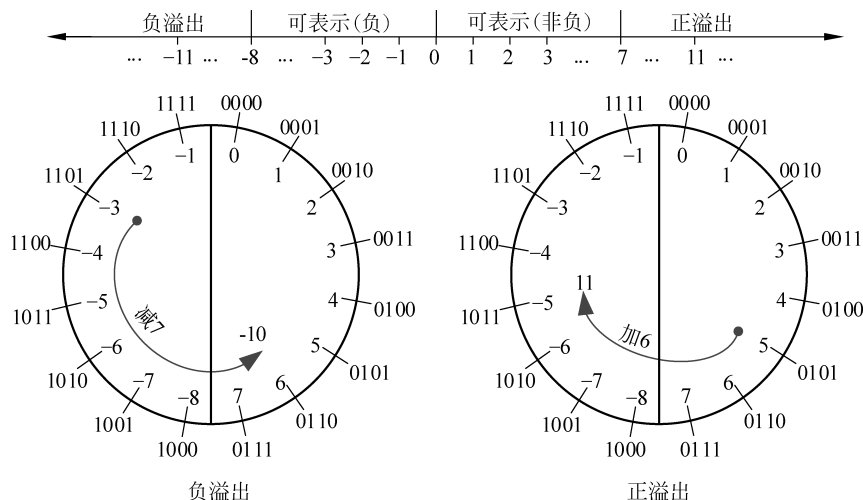
图 3-5 补码表示法的溢出
