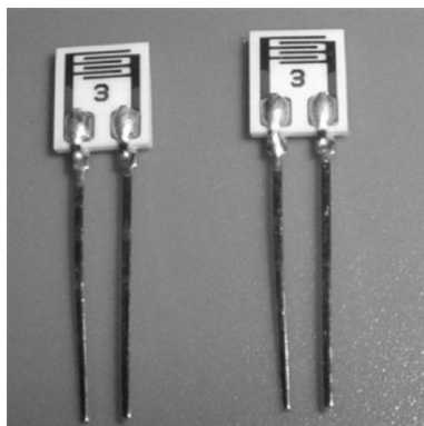
图 3-35 氯化锂湿敏电阻
