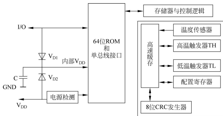
图 3-50 DS18B20 的内部结构
