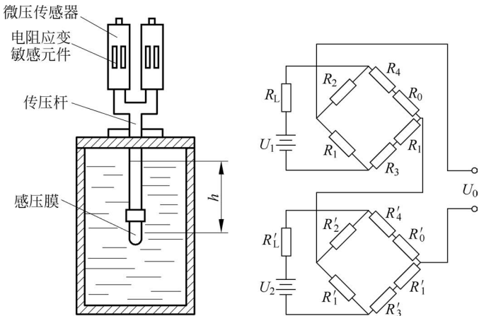
图 3-15 应变式容器内液体质量传感器的原理
