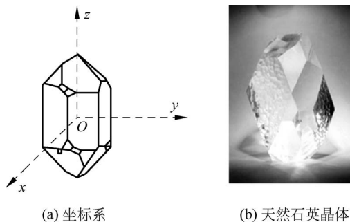
图 3-27 石英晶体及其坐标系
