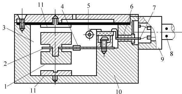
图 3-16 应变式加速度传感器的原理
