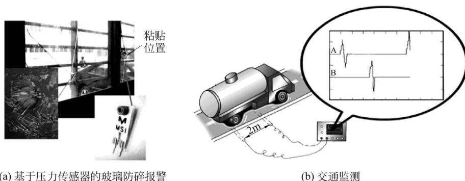
图 3-42 压力传感器的典型应用场景
