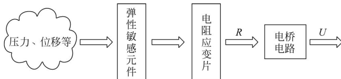
图 3-10 电阻应变式传感器的原理
