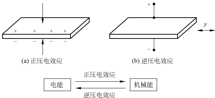
图 3-26 压电效应
