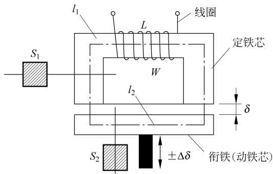
图 3-17 变磁阻式传感器的结构
