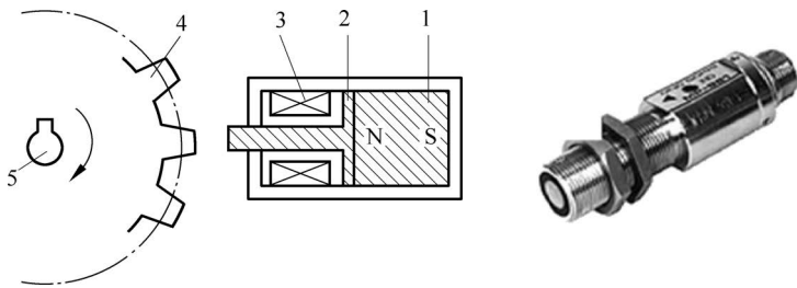
图 3-30 变磁通式磁电传感器的结构原理
