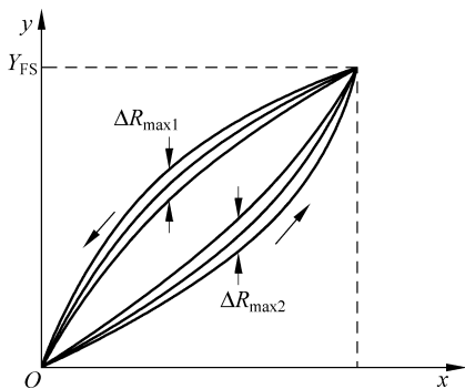
图 3-5 重复性
