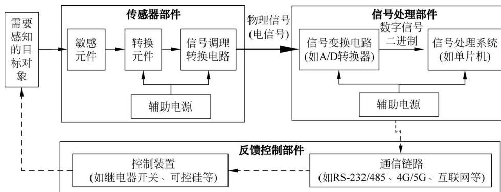
图 3-1 传感检测与反馈控制模型的功能结构
