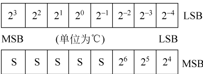
图 3-52 温度信号寄存器格式
