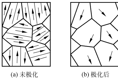
图 3-28 压电陶瓷极化图
