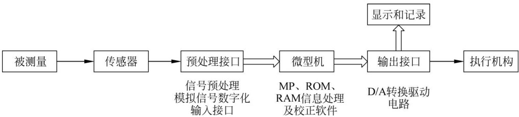
图 3-44 智能传感器构成框图
