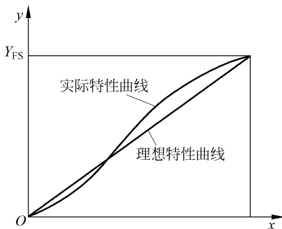
图 3-2 线性度
