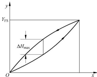
图 3-4 迟滞特性
