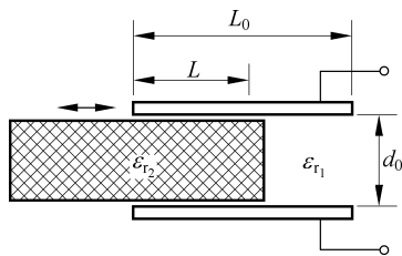
图 3-25 变介质型电容传感器
