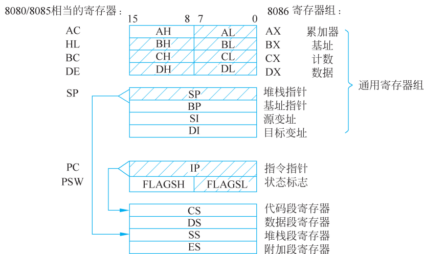
图 3.3 8086/8088 的编程结构
