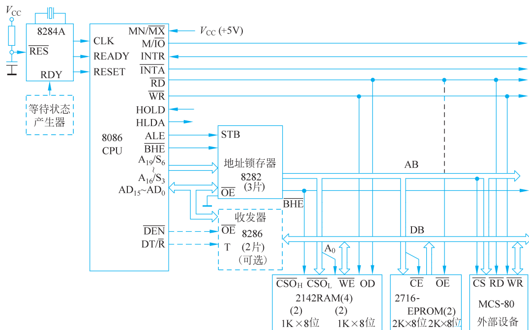
图 3.7 8086 最小方式典型的系统结构示意图
