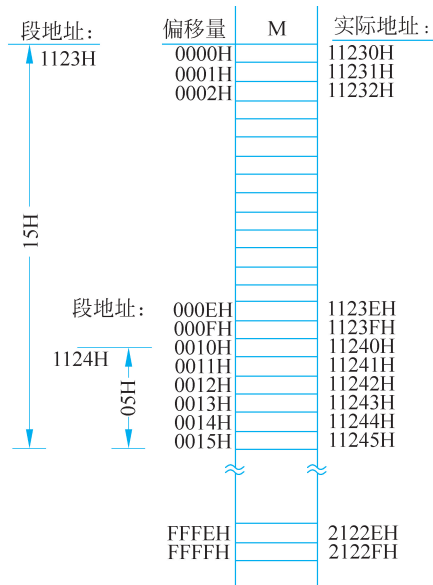
图 3.13 一个实际地址可对应多个逻辑地址
