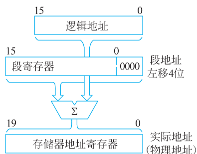
图 3.2 物理地址(实际地址)的产生过程
