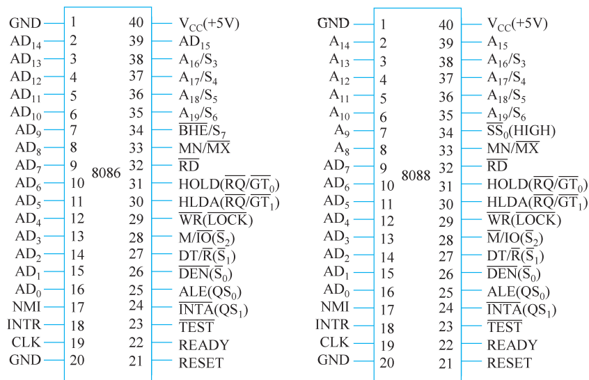
图 3.6 8086/8088 的引脚信号 (括号中为最大方式时的引脚名称)
