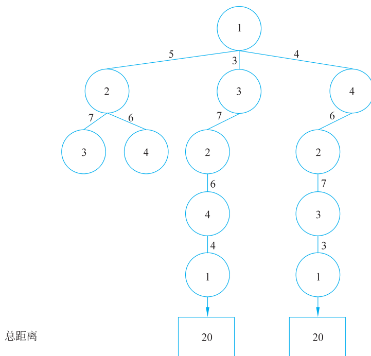
图 3.8 DFS 搜索树
