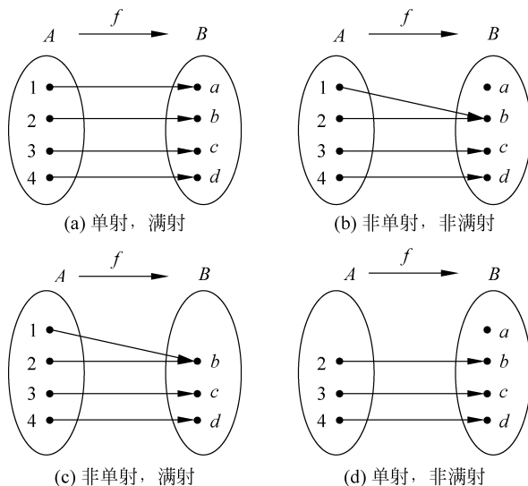
图 3.1 四种情形下的函数
