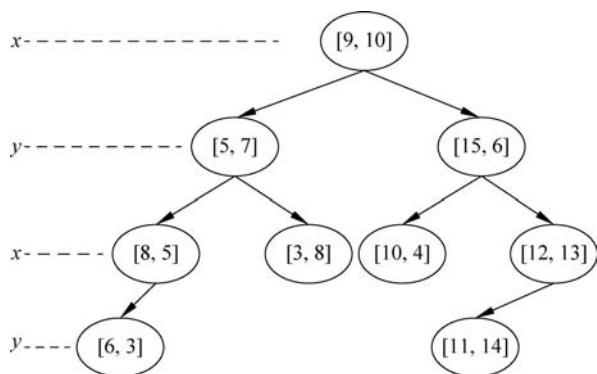
图 5-4 kd 树示例
