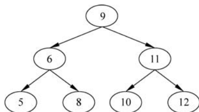
图 5-3 二叉搜索树
