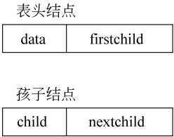
图 5-6 结点结构示意图
