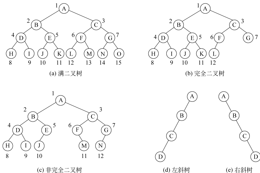
图 5-12 几种特殊二叉树
