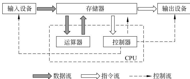
图 3.2 冯·诺依曼体系结构
