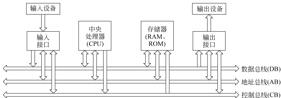
图 3.4 总线和微型计算机的基本结构
