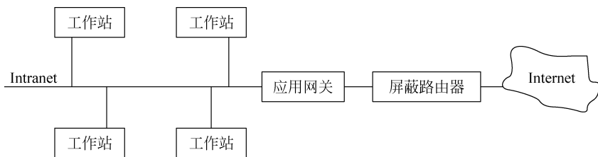
图 5-11 屏蔽主机网关示意图
