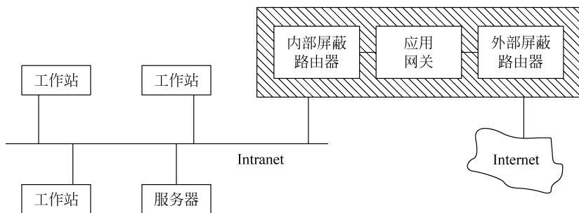
图 5-12 被屏蔽子网防火墙示意图
