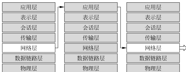
图 5-6 应用层网关防火墙
