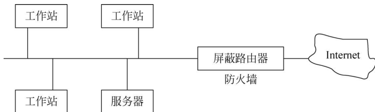
图 5-9 屏蔽路由器示意图
