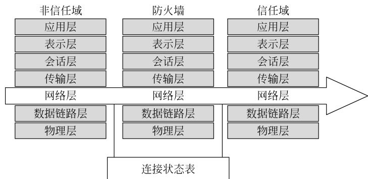
图 5-4 动态包过滤防火墙
