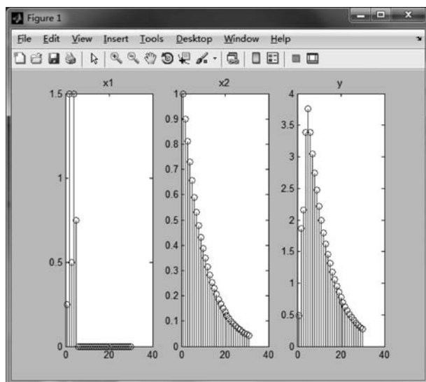
图 3-5 序列圆周积分图像
