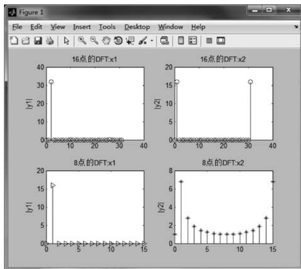
图 3-3 周期延拓序列 DFT 输出图像
