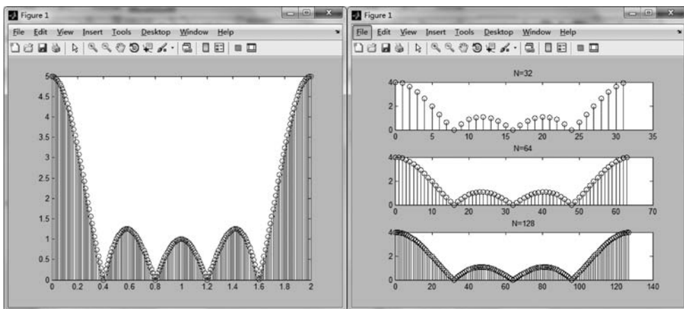
图 3-1 序列 DFT 输出
