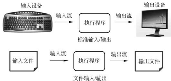
图 5-2 输入/输出流
