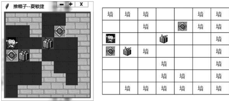
图 5-4 推箱子游戏
