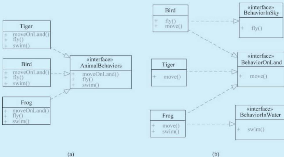
图 5-29 接口分离原则
