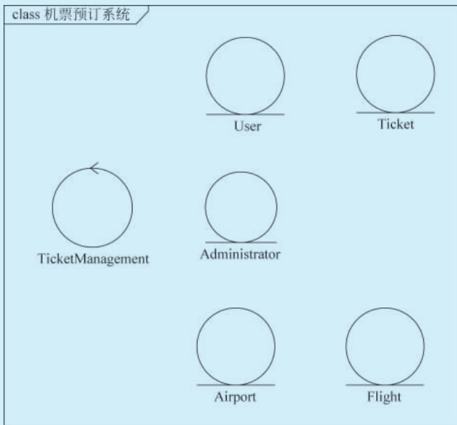
图 5-30 确定类元素
