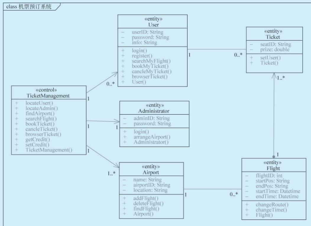
图 5-32 最终类图
