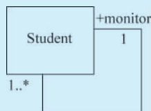
图 5-8 自关联
