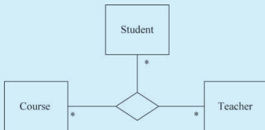
图 5-9 三元关联
