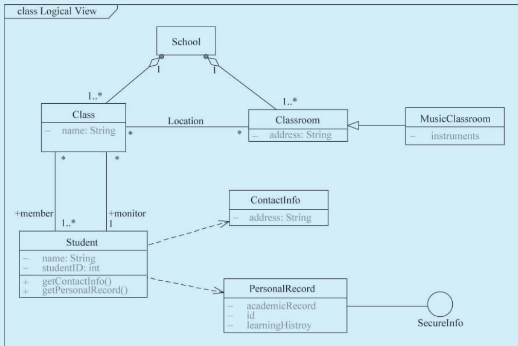
图 5-1 类图
