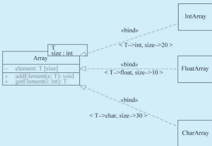
图 5-24 模板类
