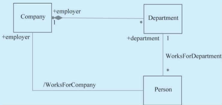
图 5-17 派生关联
