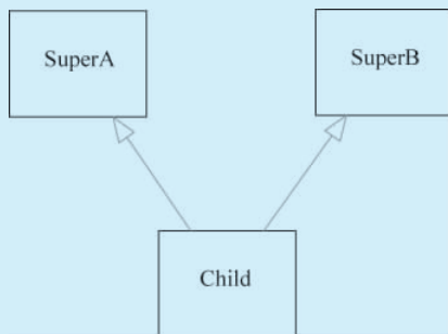
图 5-19 多重继承
