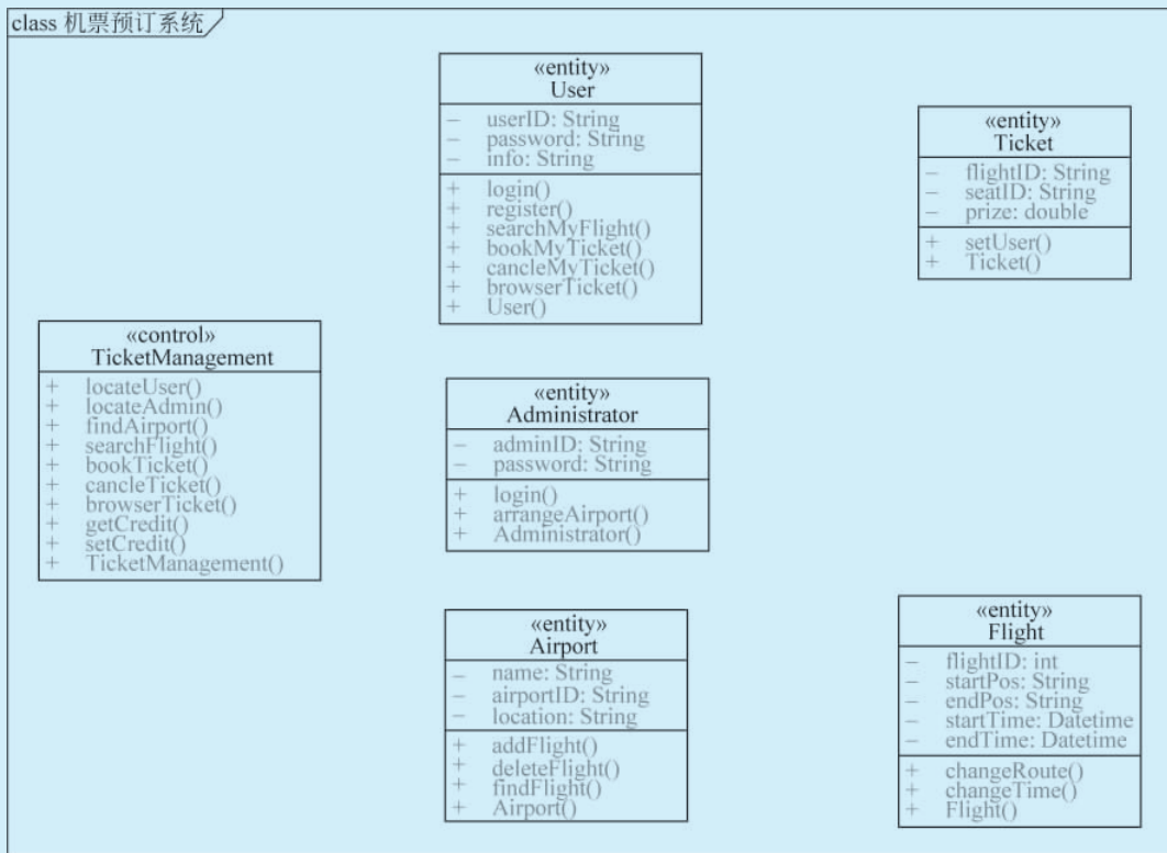
图 5-31 添加类的属性与操作
