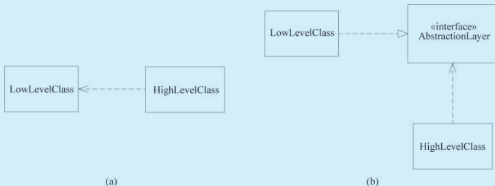
图 5-28 依赖倒置原则
