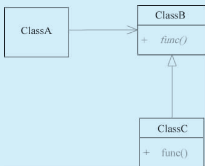
图 5-27 里氏替换原则
