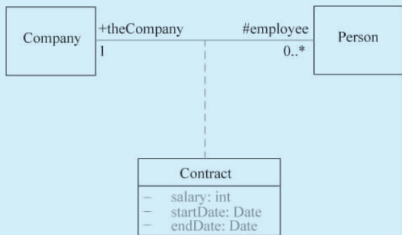
图 5-25 关联类
