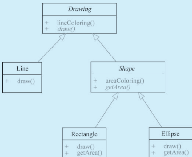
图 5-23 抽象类
