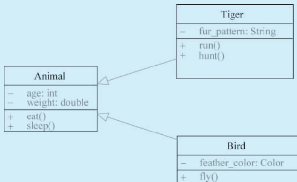
图 5-18 泛化关系
