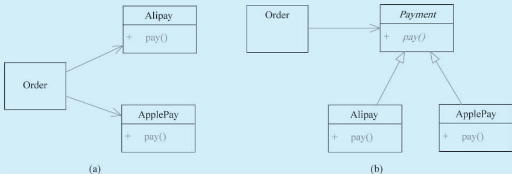
图 5-26 开闭原则
