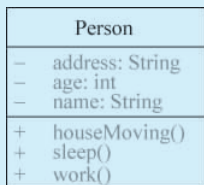
图 5-2 类
