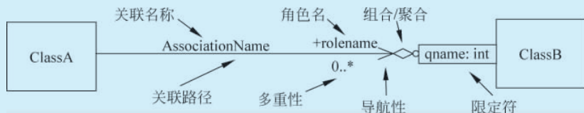
图 5-7 二元关联
