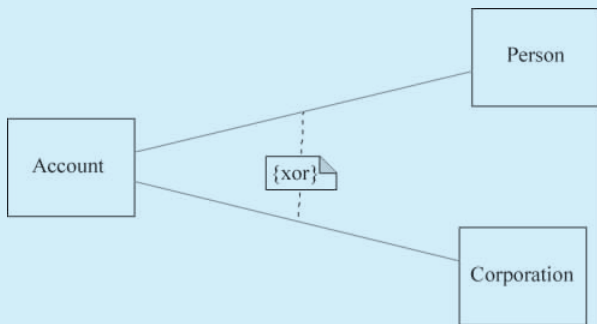
图 5-14 二元约束
