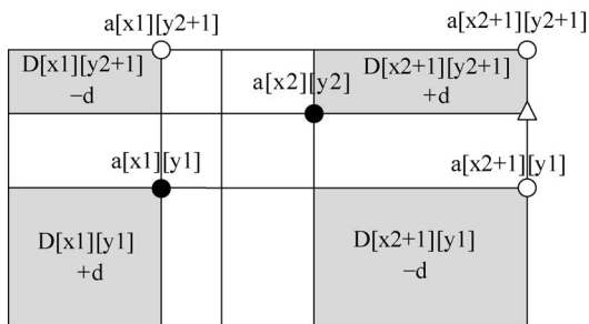
图 5.6 二维差分的区间修改
