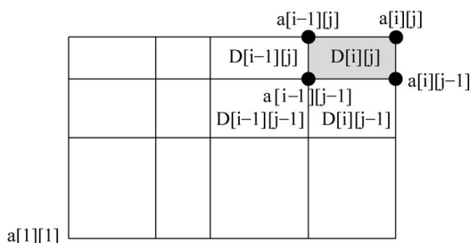
图 5.5 把每个 a[i][j] 看成总面积, 把每个 D[i][j] 看成小格子的面积
