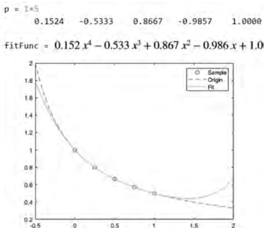
图 5-14 多项式拟合例程
