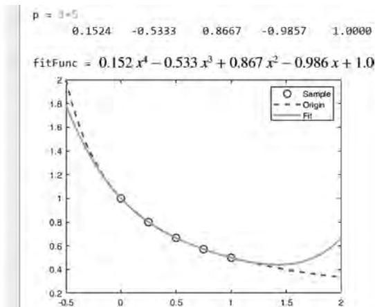
图 5-15 最小二乘拟合例程
