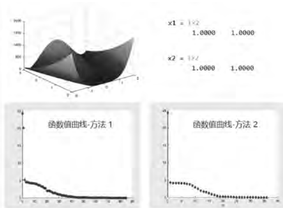
图 5-17 无约束优化例题
