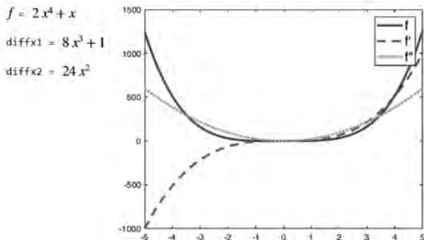
图 5-7 导数例程
