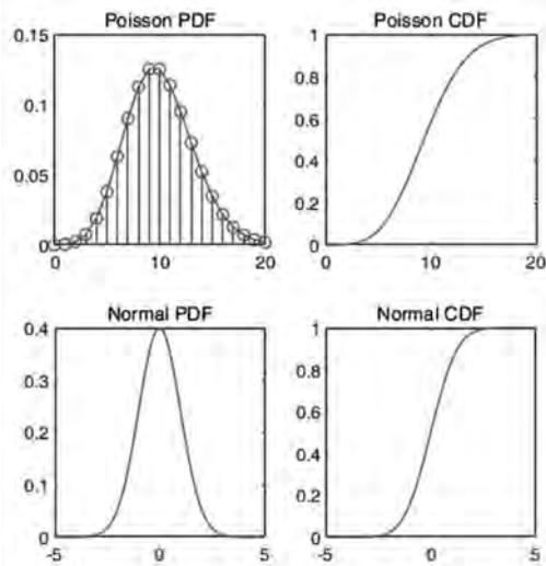
图 5-35 概率分布与概率密度例程
