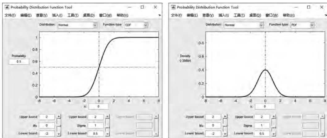
图 5-36 概率分布函数 App
