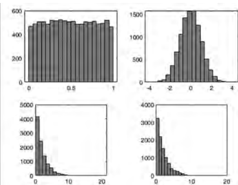
图 5-37 伪随机数例程
