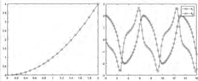
图 5-22 常微分方程数值解例程
