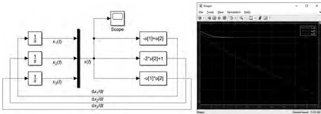
图 5-23 微分方程 Simulink 求解
