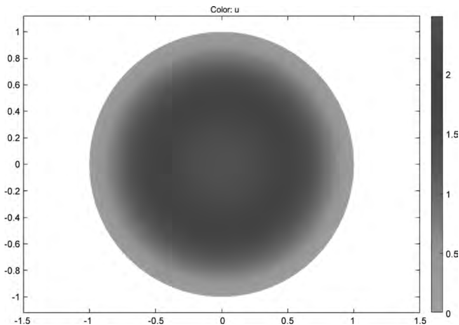
图 5-30 方程解的云图
