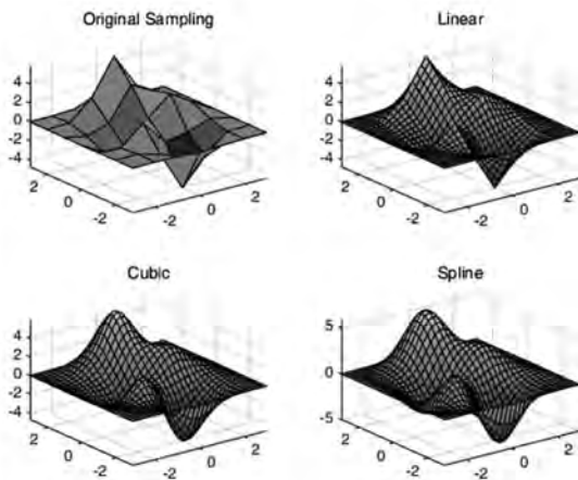
图 5-12 二维网格数据插值例程
