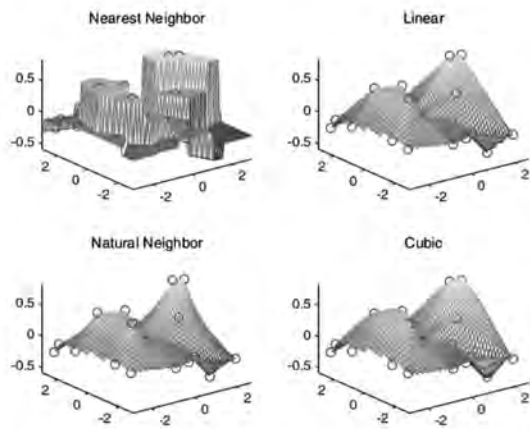
图 5-13 二维一般数据插值例题
