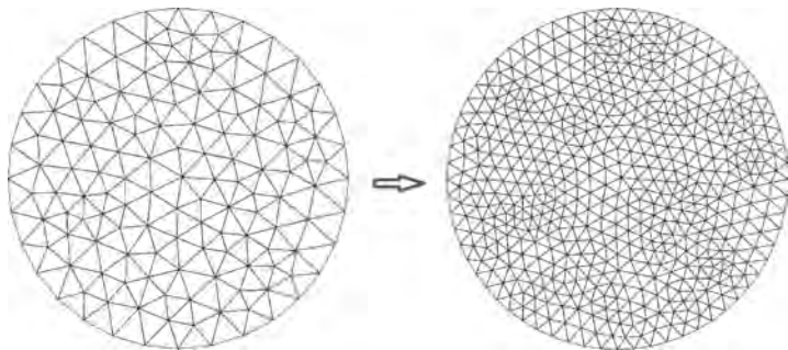
图 5-29 网格细化设置
