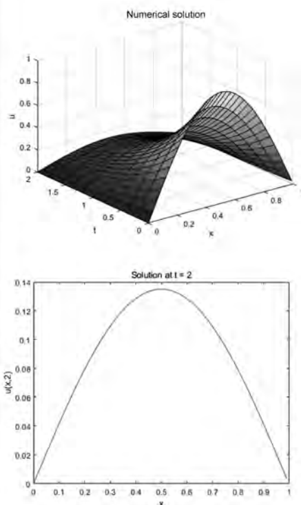
图 5-24 抛物-椭圆形偏微分方程例程
