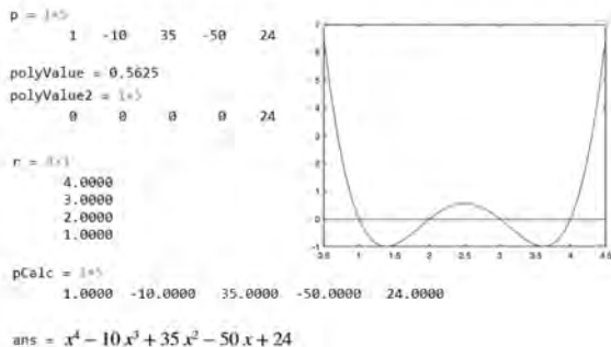
图 5-2 多项式例题
