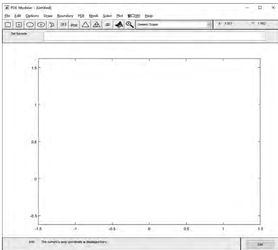
图 5-25 PDE 工具箱界面
