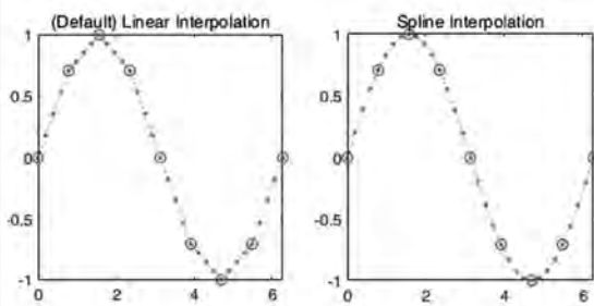
图 5-11 一维插值例程
