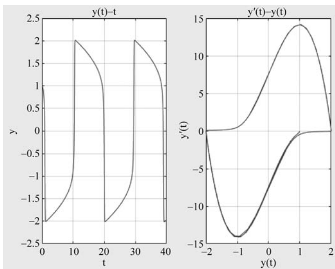
图 3-6 Van Der Pol 微分方程解
