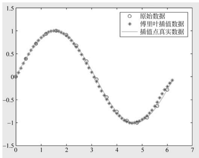
图 3-1 一维快速傅里叶插值及比较
