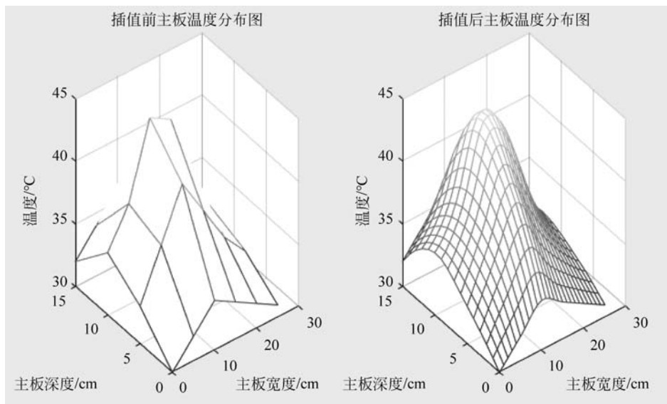
图 3-3 插值前后主板温度分布图
