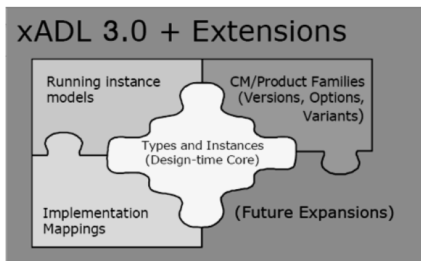
图 5-5 xADL 3.0 的结构
