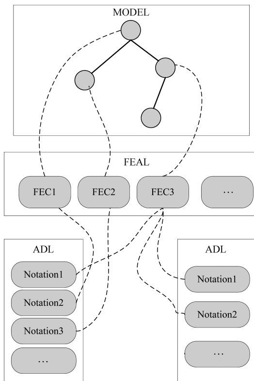
图 5-4 ADL、FEAL、MODEL 的关系
