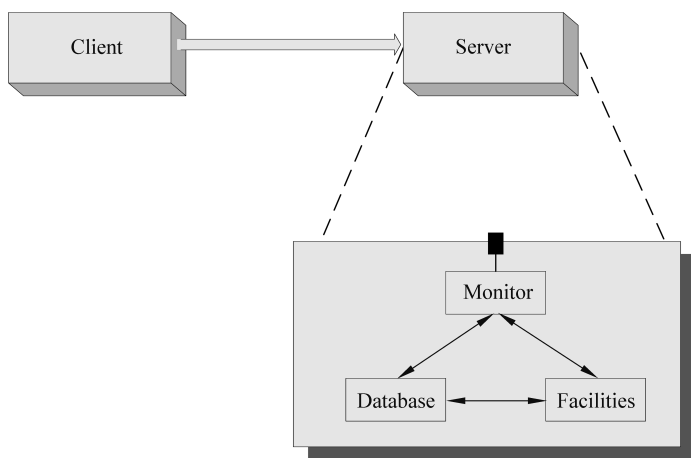
图 5-1 层次构件
