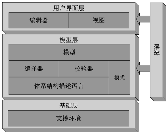
图 5-2 原型框架
