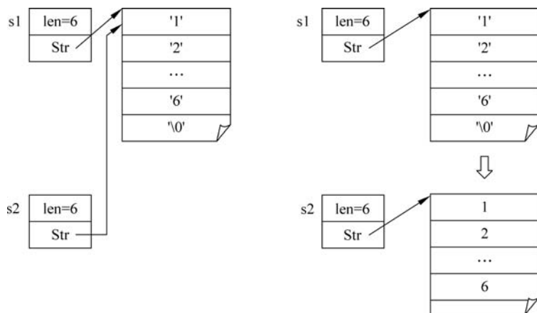
执行“String s2=s1;”进行浅拷贝
