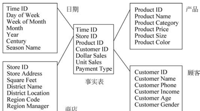
图 3.8 某公司销售数据仓库的星型模型
