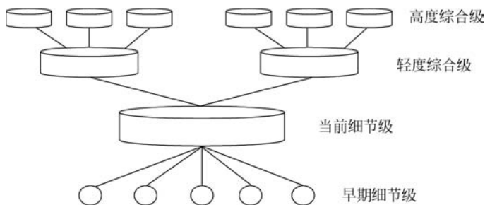
图 3.6 典型数据仓库的粒度结构
