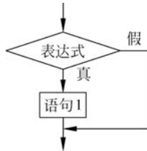
图 3-1 if 语句的流程
