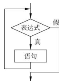
图 3-4 while 语句的流程
