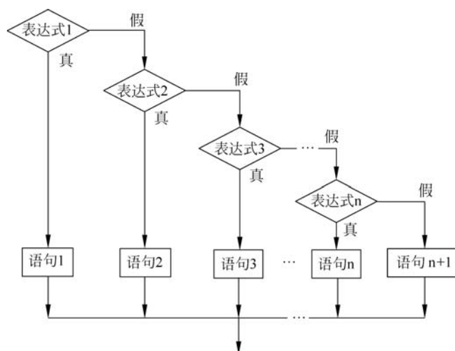
图 3-3 if...elif...else 语句的流程
