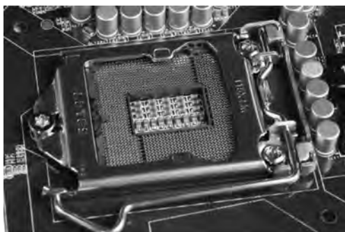
图 3-11 CPU 插槽
