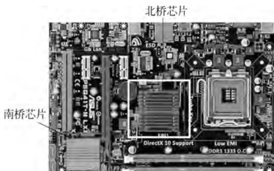
图 3-9 南北桥芯片
