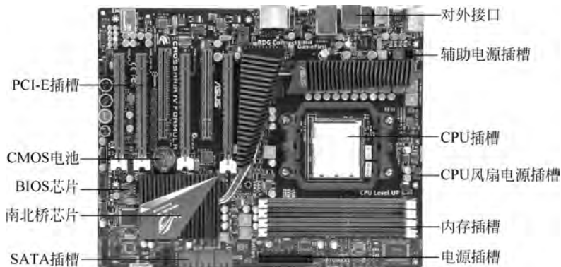
图 3-1 主板示意图
