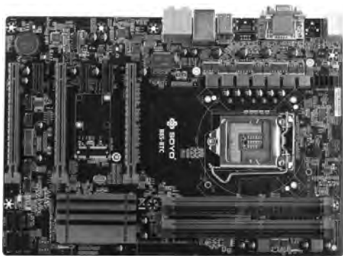
图 3-2 ATX 主板
