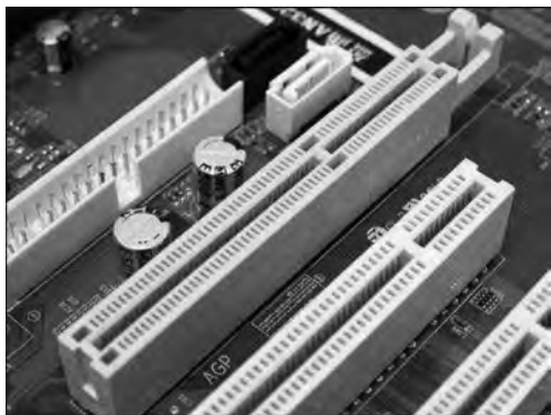
图 3-15 AGP 插槽
