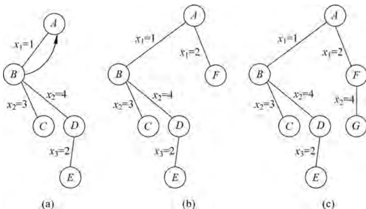
图 5-10 搜索过程 3
