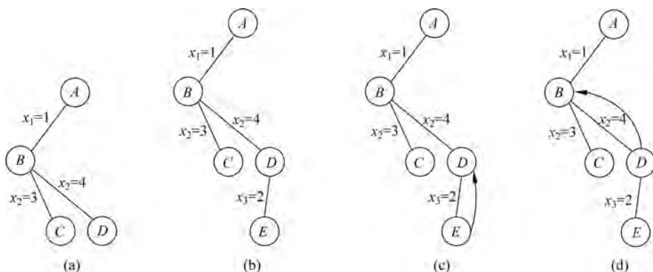
图 5-9 搜索过程 2
