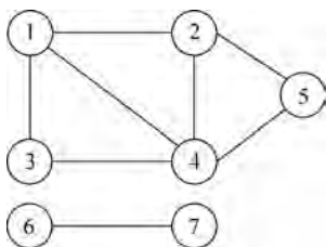
图 5-4 无向图
