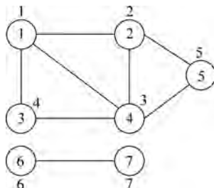
图 5-5 搜索顺序
