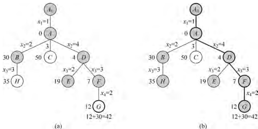
图 5-71 搜索过程 3
