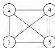
图 5-25 最大团
