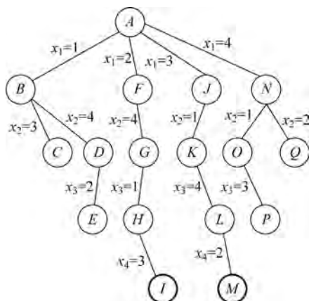
图 5-13 搜索过程 6
