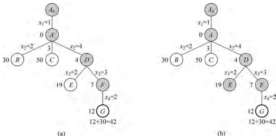
图 5-70 搜索过程 2
