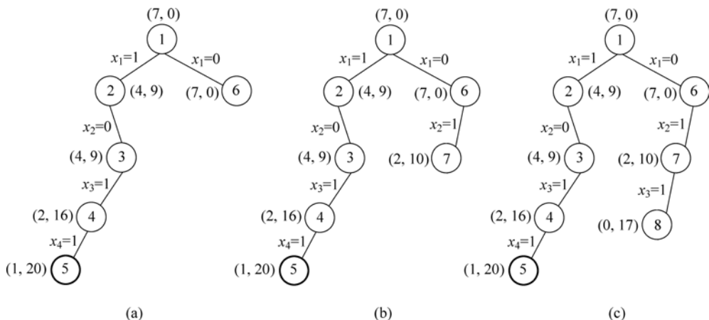
图 5-19 搜索过程 3
