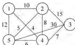
图 5-35 无向带权图
