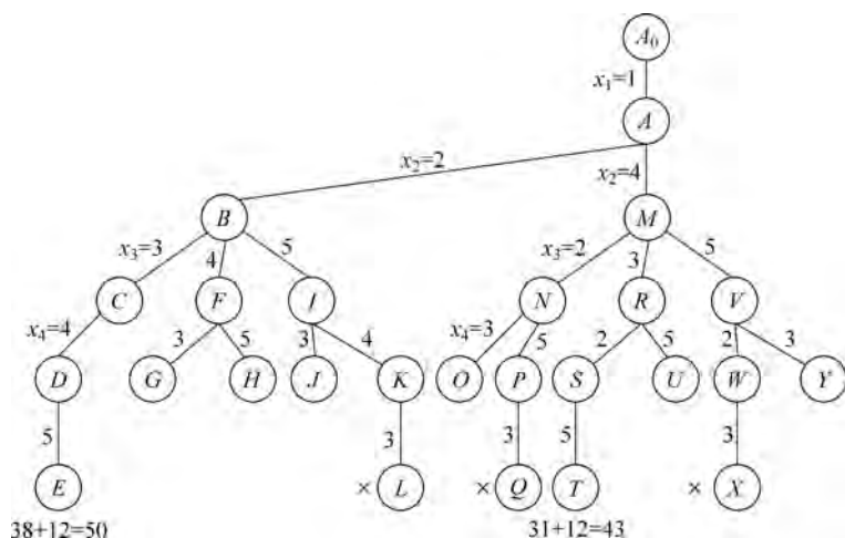
图 5-39 搜索过程 4
