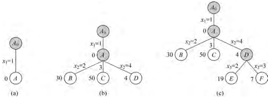
图 5-69 搜索过程 1
