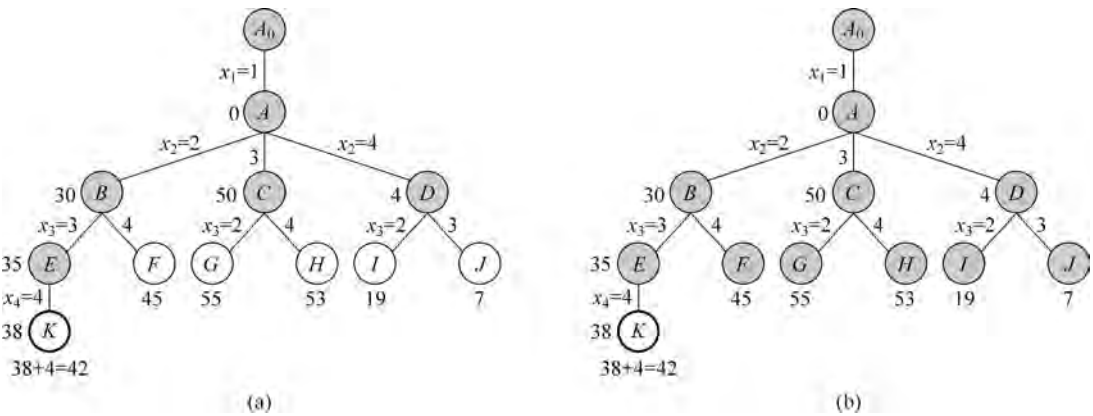
图 5-68 搜索过程 3
