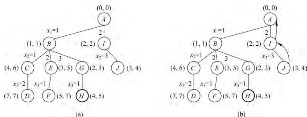
图 5-53 搜索过程 5
