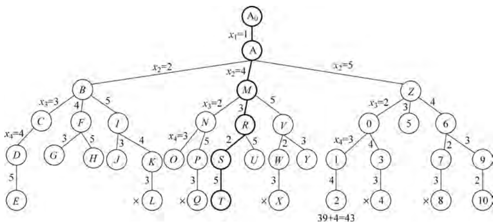
图 5-40 搜索过程 5
