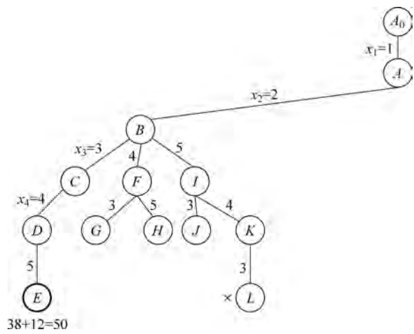
图 5-38 搜索过程 3
