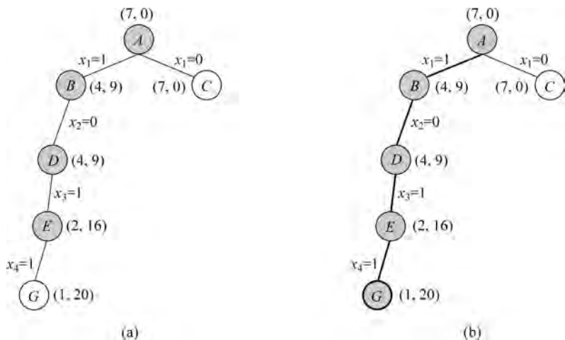
图 5-64 搜索过程 2
