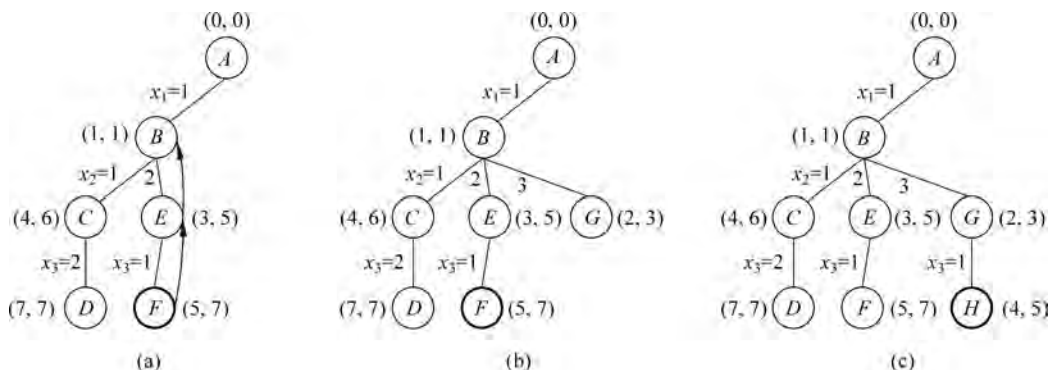
图 5-51 搜索过程 3
