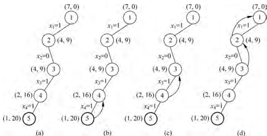
图 5-18 搜索过程 2
