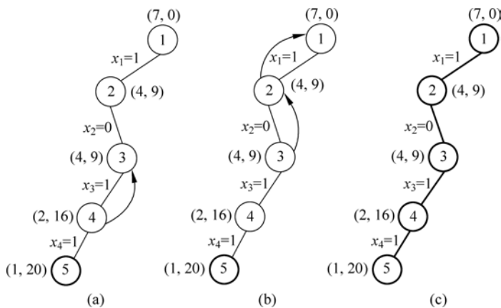
图 5-22 搜索过程
