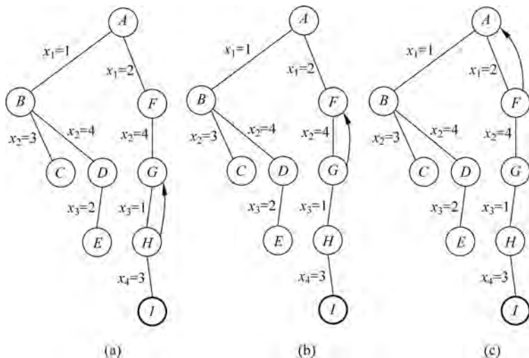
图 5-12 搜索过程 5
