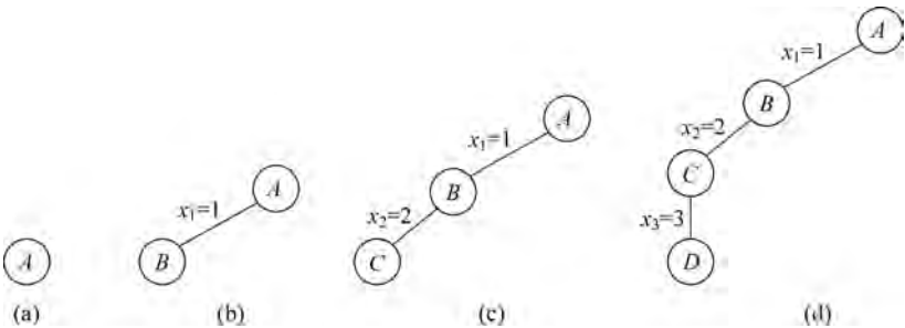
图 5-43 搜索过程 1
