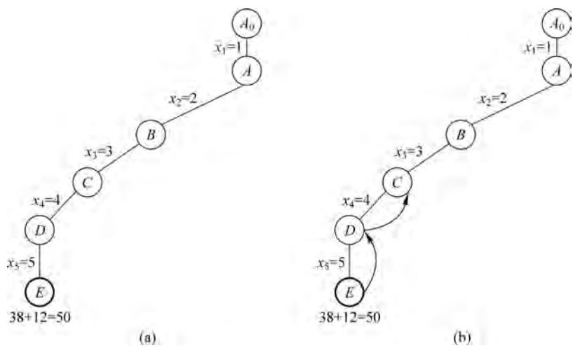
图 5-37 搜索过程 2
