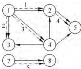
图 5-56 搜索顺序
