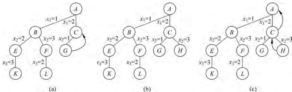
图 5-30 搜索过程 4
