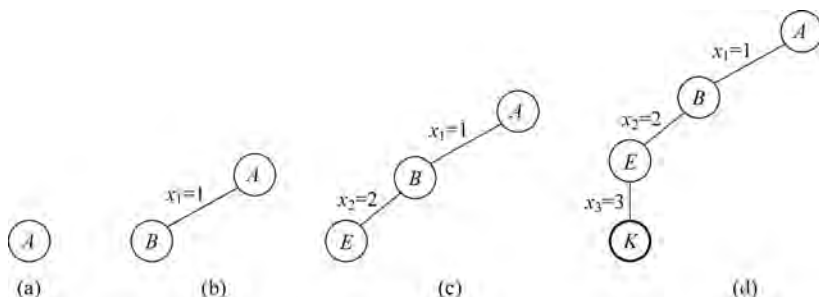
图 5-27 搜索过程 1
