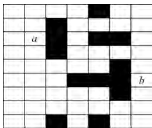
图 5-73 9×7 阵列
