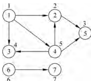
图 5-3 搜索顺序
