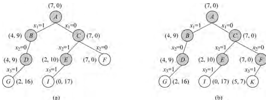
图 5-61 搜索过程 3
