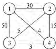
图 5-65 无向连通图
