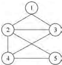
图 5-42 无向连通图
