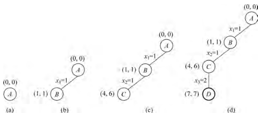
图 5-49 搜索过程 1
