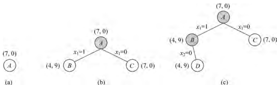
图 5-59 搜索过程 1
