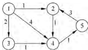
图 5-1 有向带权图
