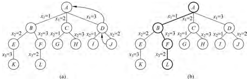
图 5-33 搜索过程 7
