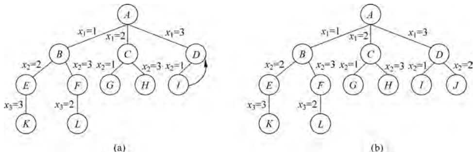
图 5-32 搜索过程 6
