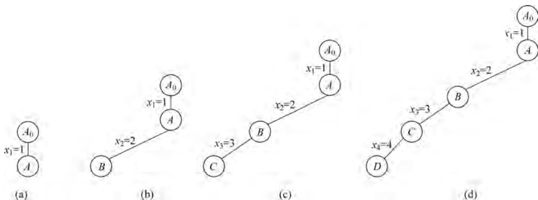
图 5-36 搜索过程 1
