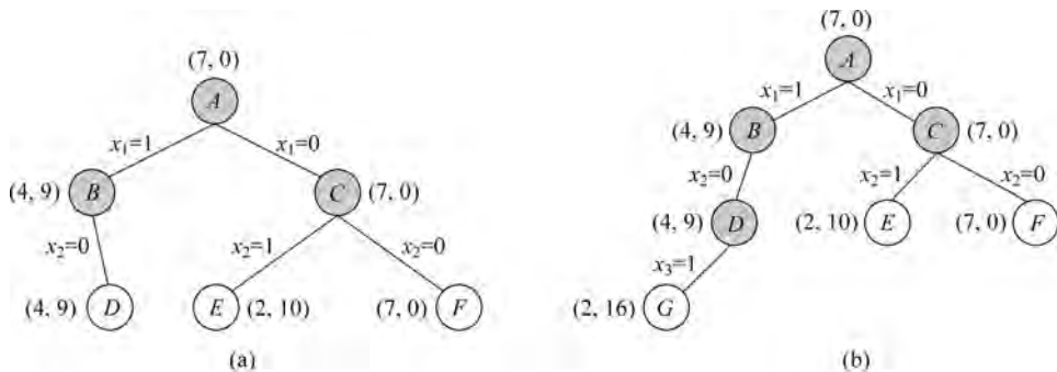
图 5-60 搜索过程 2
