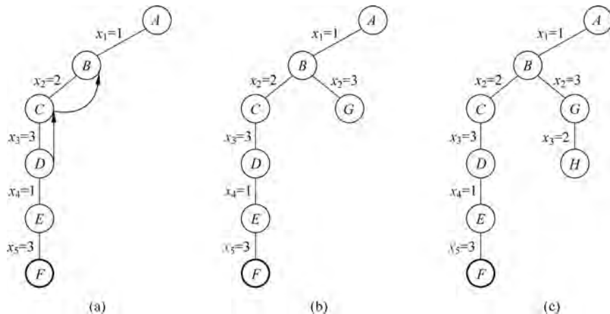
图 5-45 搜索过程 3
