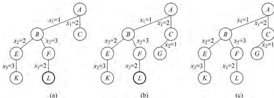
图 5-29 搜索过程 3
