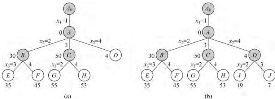
图 5-67 搜索过程 2
