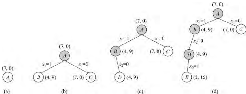
图 5-63 搜索过程 1
