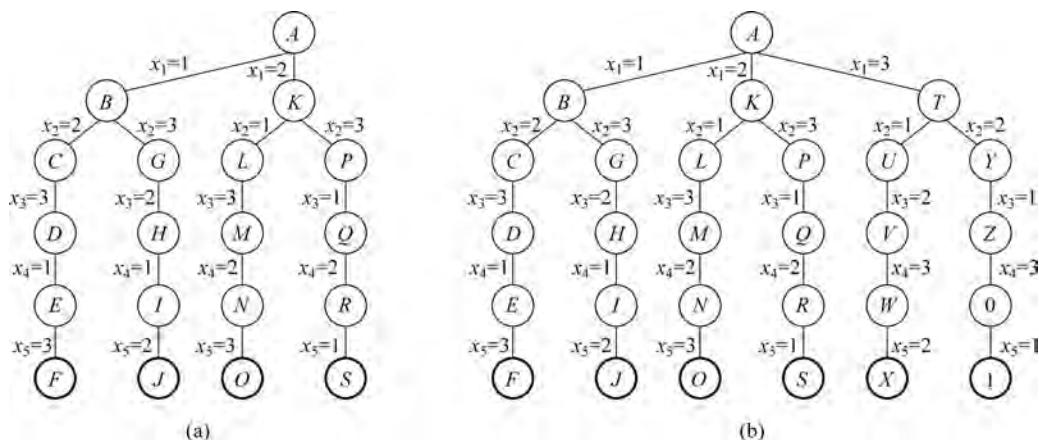
图 5-48 搜索过程 6
