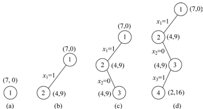
图 5-17 搜索过程 1
