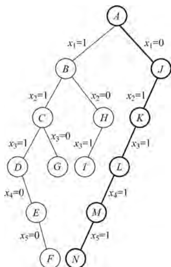
图 5-24 搜索树
