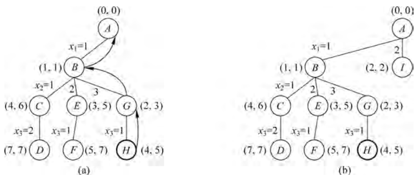
图 5-52 搜索过程 4
