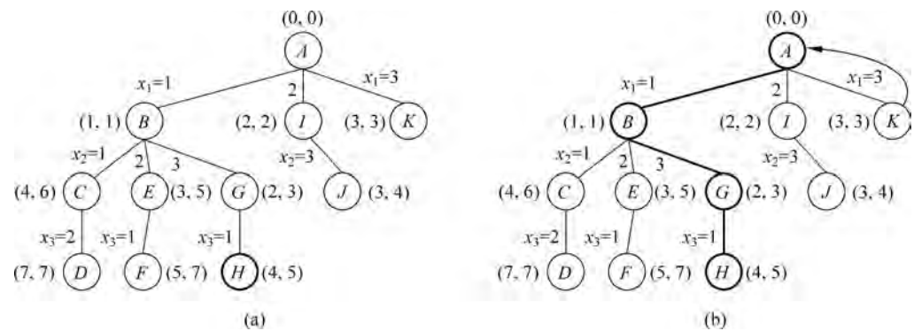
图 5-54 搜索过程 6
