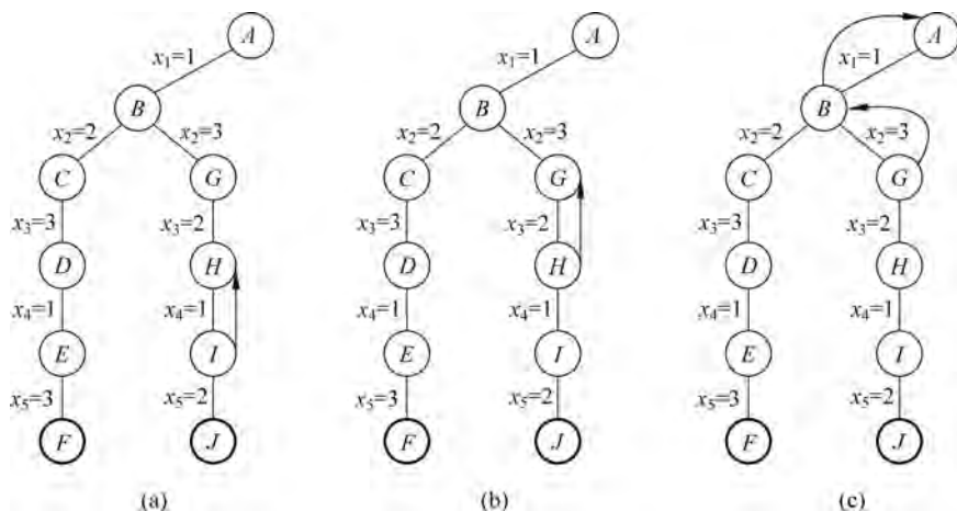
图 5-47 搜索过程 5
