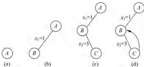
图 5-8 搜索过程 1
