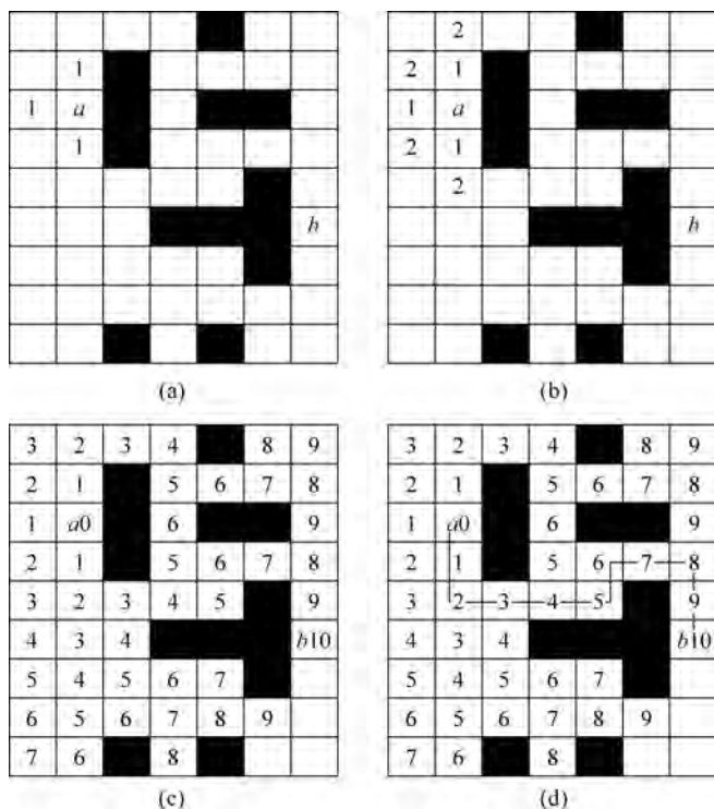
图 5-74 构造最优解
