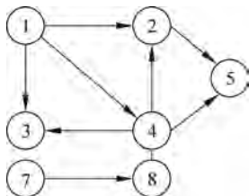
图 5-55 有向图
