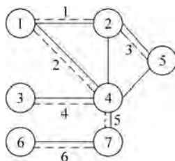
图 5-58 搜索顺序
