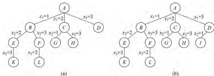
图 5-31 搜索过程 5
