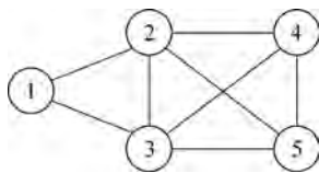
图 5-23 无向图
