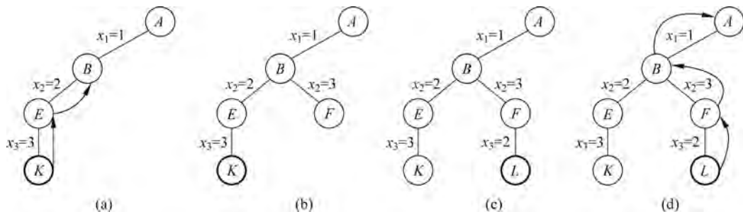
图 5-28 搜索过程 2
