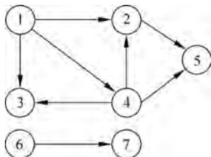
图 5-2 有向图
