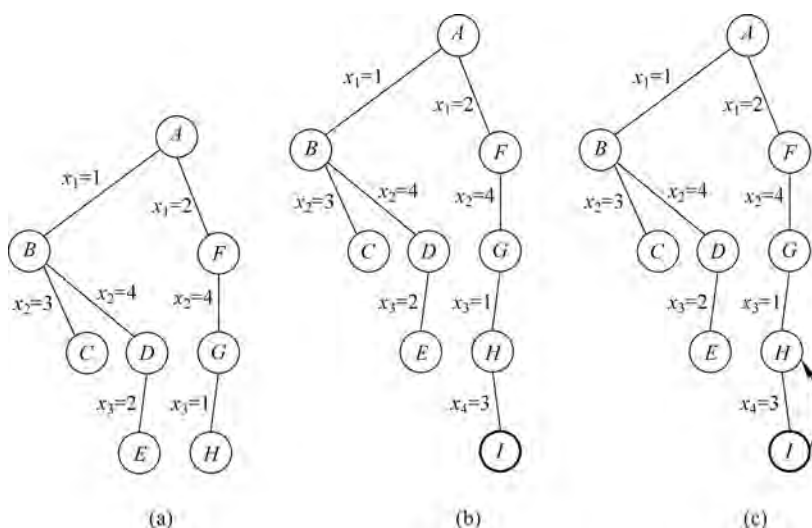
图 5-11 搜索过程 4
