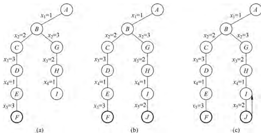
图 5-46 搜索过程 4
