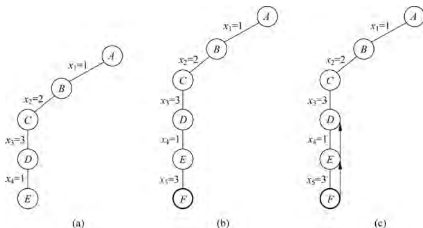
图 5-44 搜索过程 2
