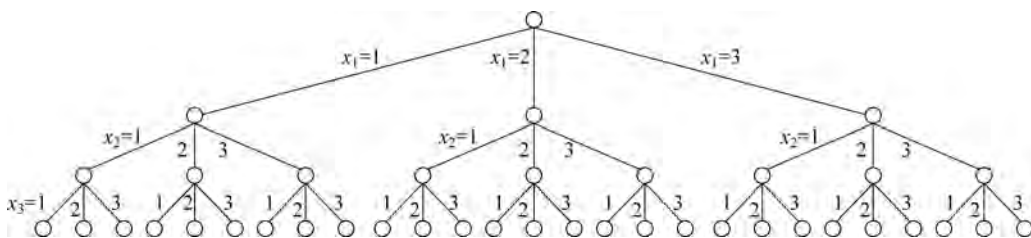
图 5-41 满 3 叉树
