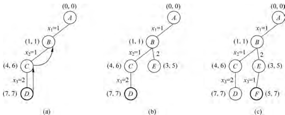
图 5-50 搜索过程 2
