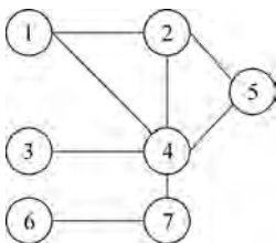
图 5-57 无向图
