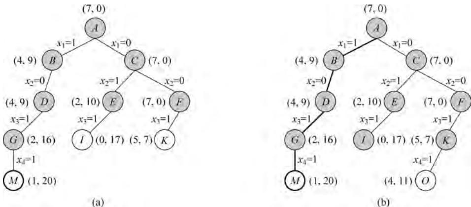
图 5-62 搜索过程 4
