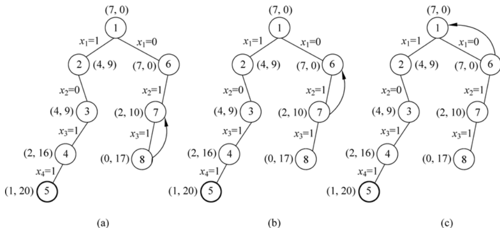
图 5-20 搜索过程 4
