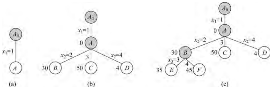
图 5-66 搜索过程 1
