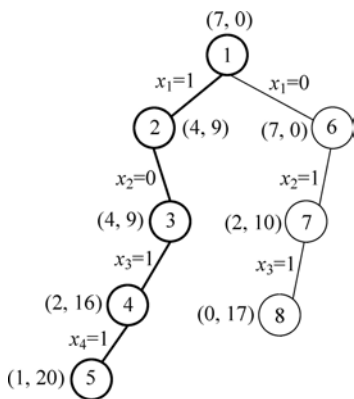
图 5-21 搜索过程 5
