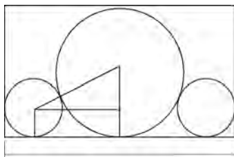
图 5-76 题 5-6
