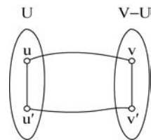
图 3-41 含有 (u, v) 的回路
