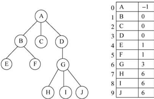
图 3-13 树的双亲表示法
