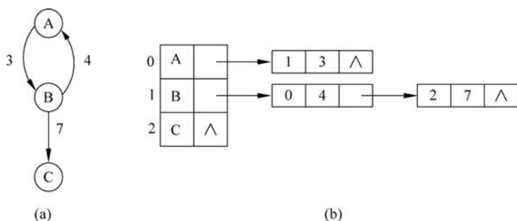
图 3-35 有向带权图及其邻接表
