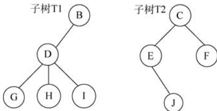
图 3-2 两棵子树
