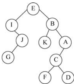
图 3-54 二叉树(2)
