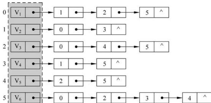
图 3-60 邻接表(1)
