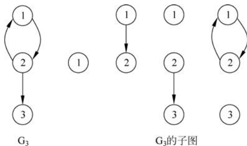
图 3-31 图与子图
