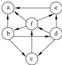
图 3-57 有向图(1)
