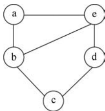
图 3-55 无向图(1)
