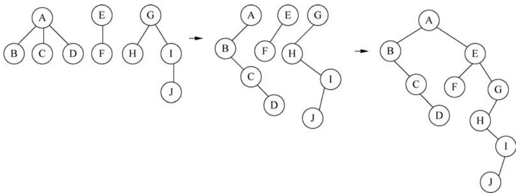
图 3-21 森林转换为二叉树的过程
