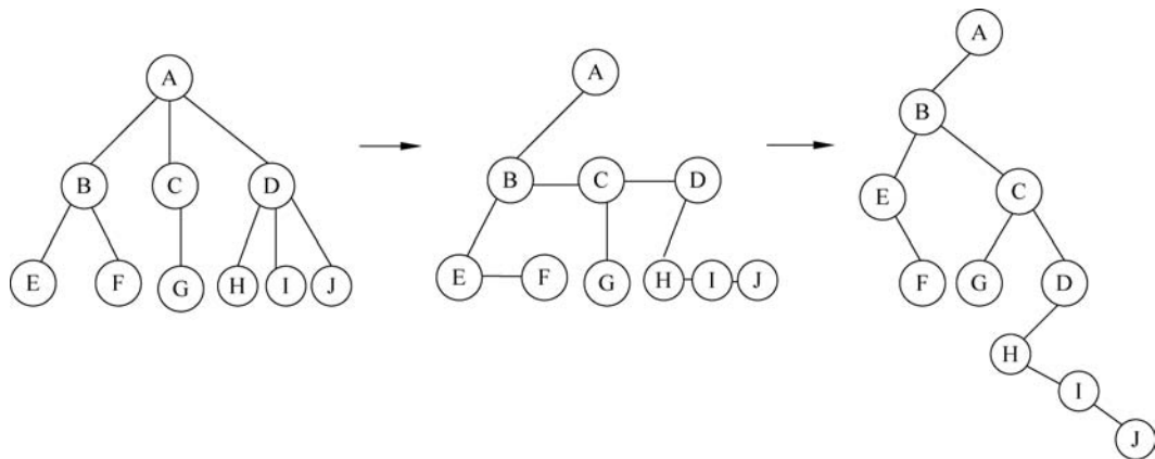
图 3-19 树转为二叉树的过程
