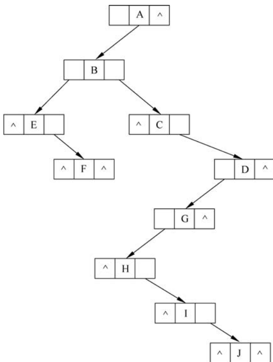
图 3-18 树的孩子兄弟表示法
