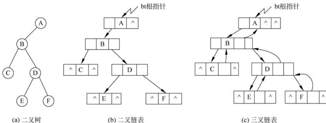
图 3-10 链表存储结构
