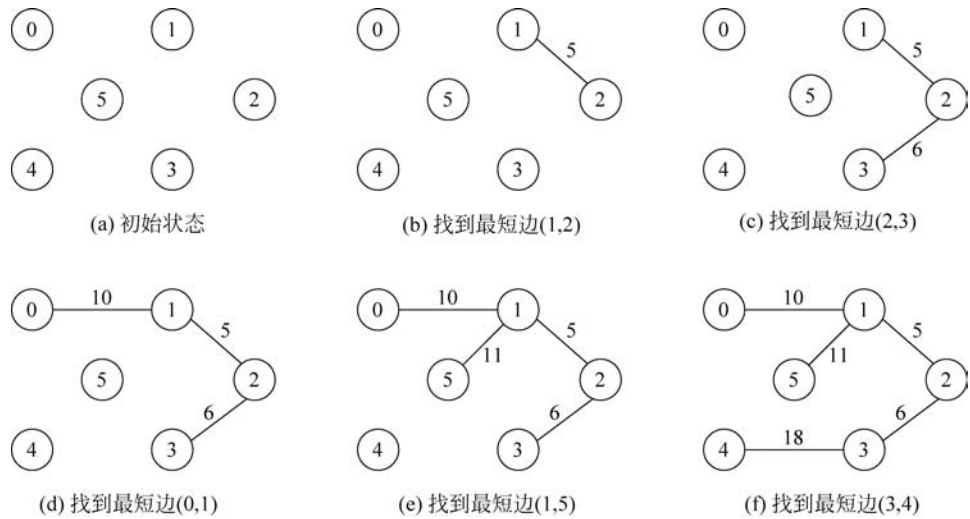
图 3-44 Kruskal 算法构造最小生成树的过程
