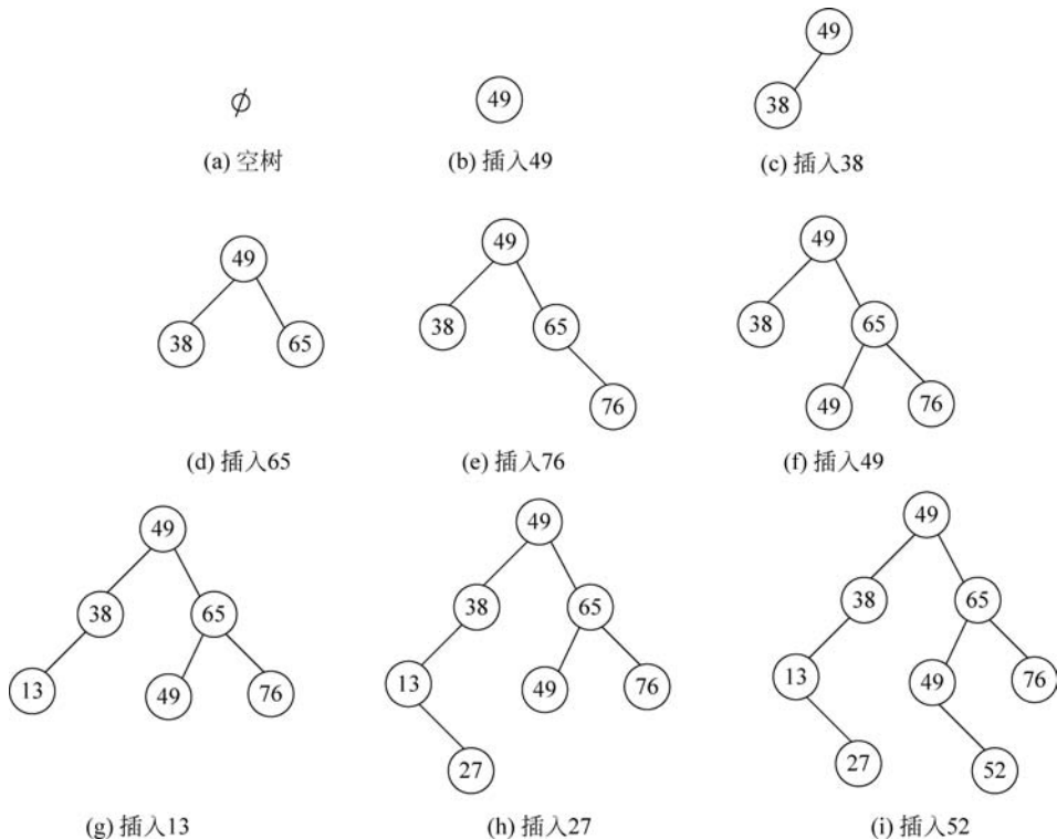
图 3-28 由关键字序列生成二叉排序树的过程
