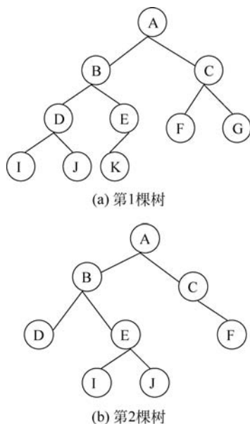
图 3-51 两棵二叉树
