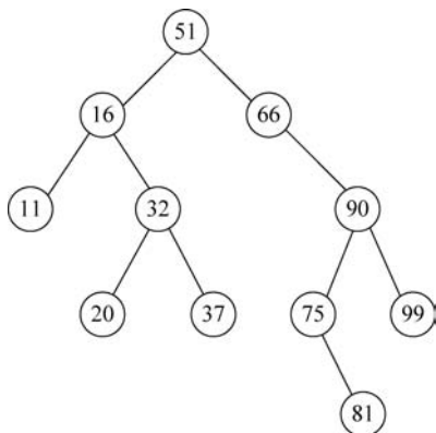
图 3-27 二叉排序树
