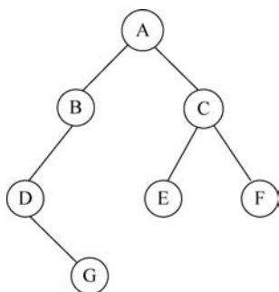
图 3-12 二叉树
