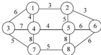
图 3-56 无向图(2)
