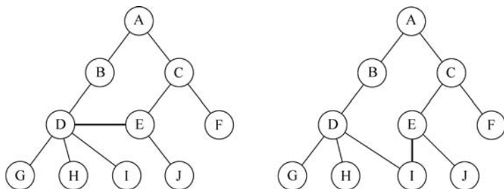
图 3-3 非树的表示
