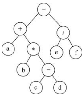
图 3-53 二叉树(1)
