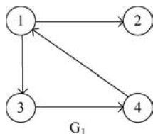
图 3-29 有向图示例
