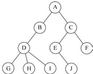
图 3-1 一般的树
