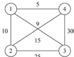
图 3-32 网(带权图)
