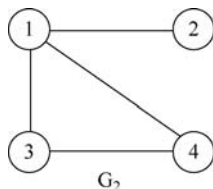
图 3-30 无向图示例
