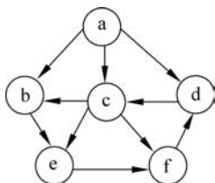
图 3-59 有向图(3)
