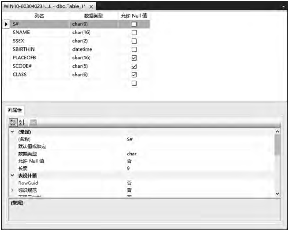
图 3.28 设计好的“学生表”S
