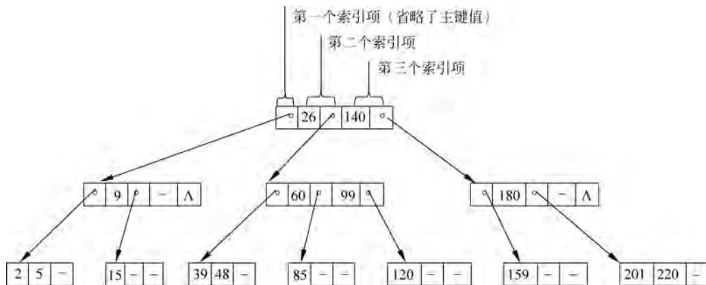
图 3.40 图 3.39 中多级索引的 B-树
