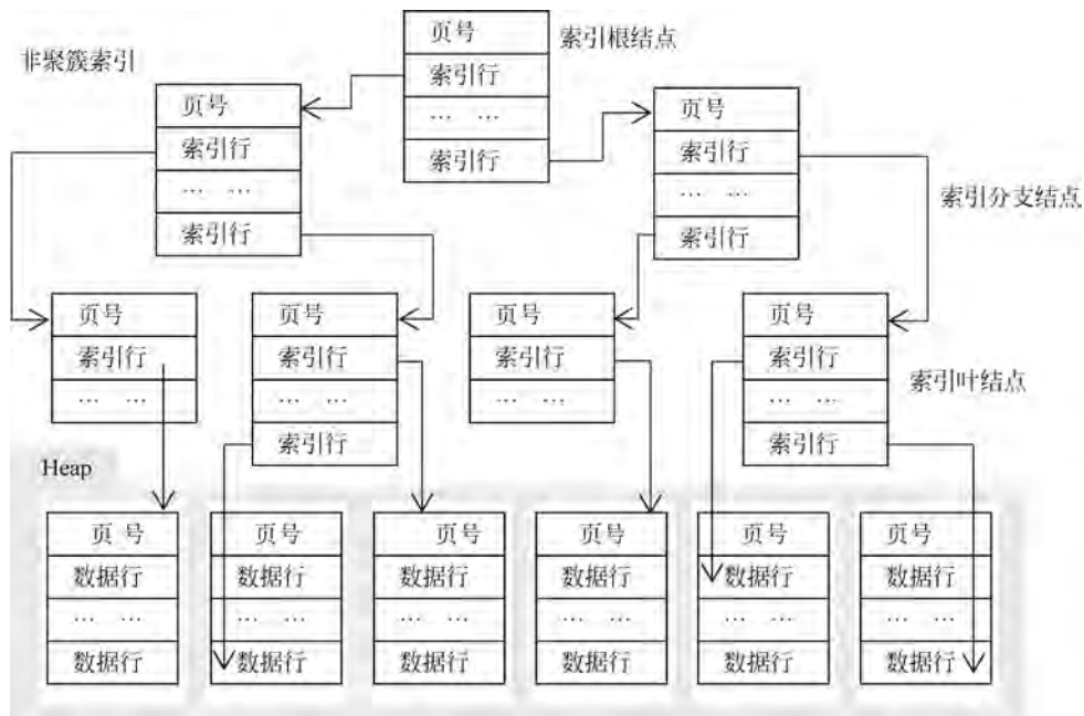
图 3.42 非聚集索引的结构示意图
