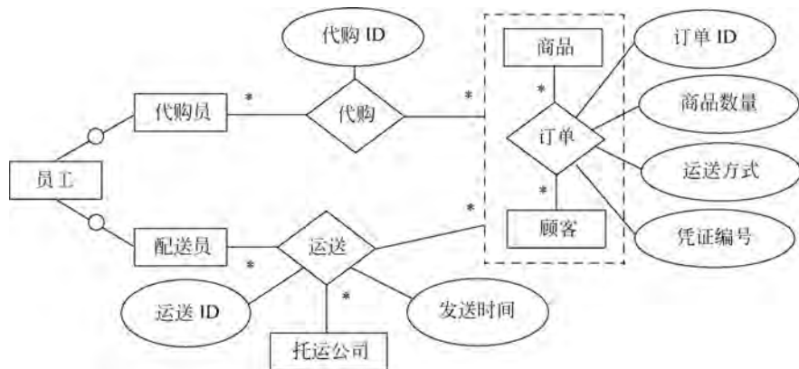
图 3.16 组合实体集 E-R 图示例
