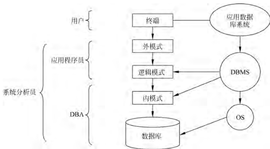
图 3.2 数据库应用系统的视图级别模型
