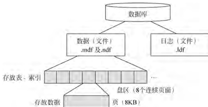
图 3.21 SQL Server 数据库的存储结构
