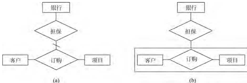
图 3.15 担保-订购关系的 E-R 图
