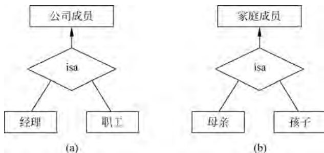
图 3.13 图 3.10(a)和图 3.10(b)的递归联系的 isa 联系 E-R 图表示
