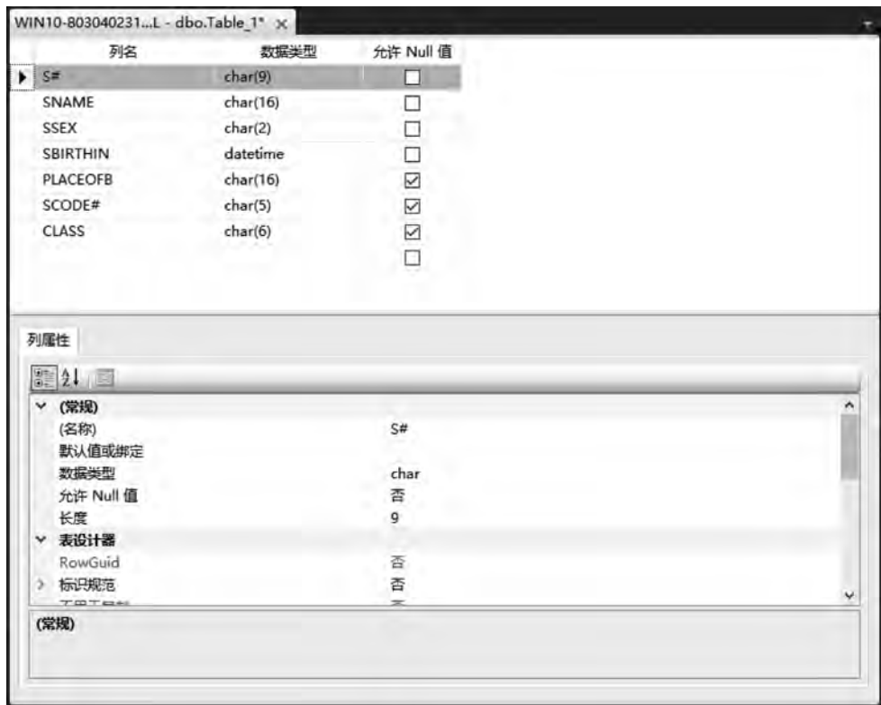
图 3.30 “设置主键”的过程——S# 为主键
