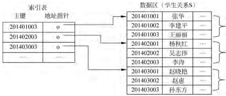
图 3.38 学生关系的稀疏索引方式
