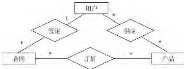
图 3.11 冗余联系示例
