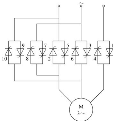
图 5-5 采用晶闸管反并联的异步电动机可逆和制动电路
