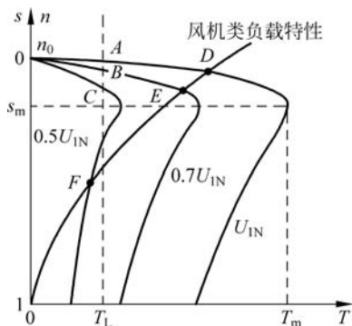
图 5-2 异步电动机改变定子电压时的机械特性
