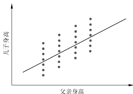
图 5-1 父亲身高与儿子身高的关系
