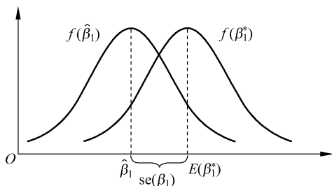
图 5-6 估计量的分布及其偏移
