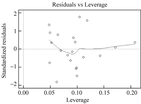
图 5-5 标准化残差对杠杆值的散点图
