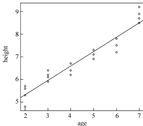
图 5-3 线性回归拟合结果
