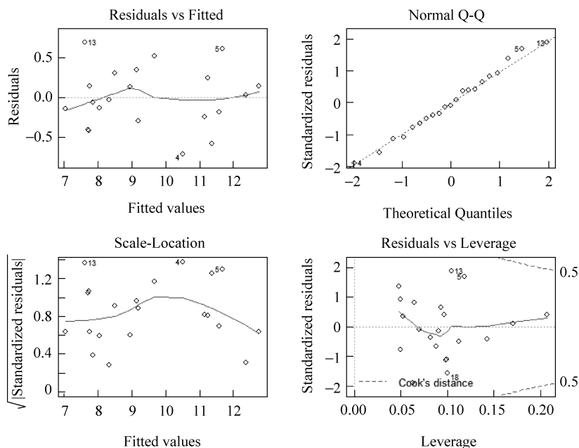
图 5-4 线性回归模型的诊断信息
