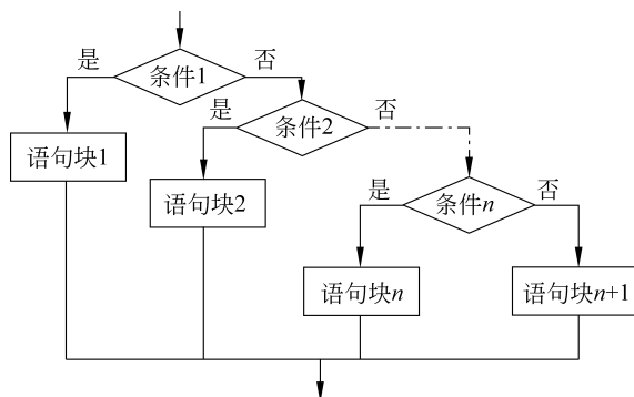
图 3.6 多分支结构的程序流程图
