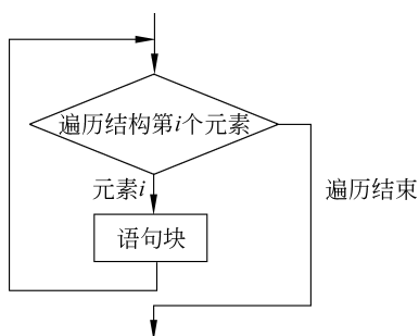
图 3.8 遍历循环结构的程序流程图
