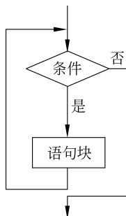
图 3.7 条件循环结构的程序流程图
