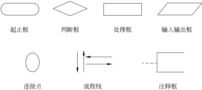
图 3.1 程序流程图的构成元素
